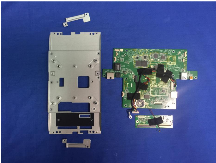
(4) EUT Photo
