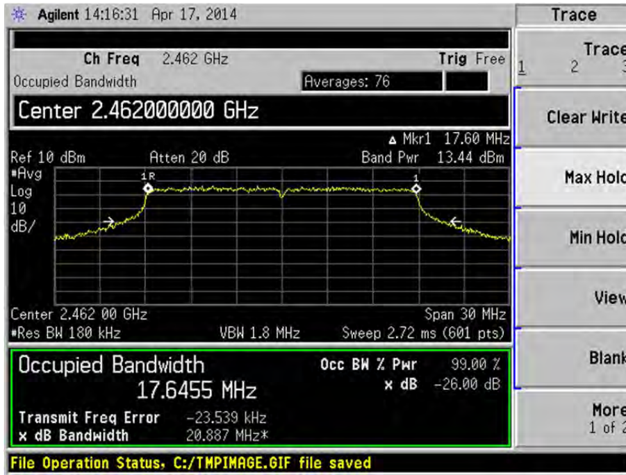
802.11 n-HT20 (Channel 11)
