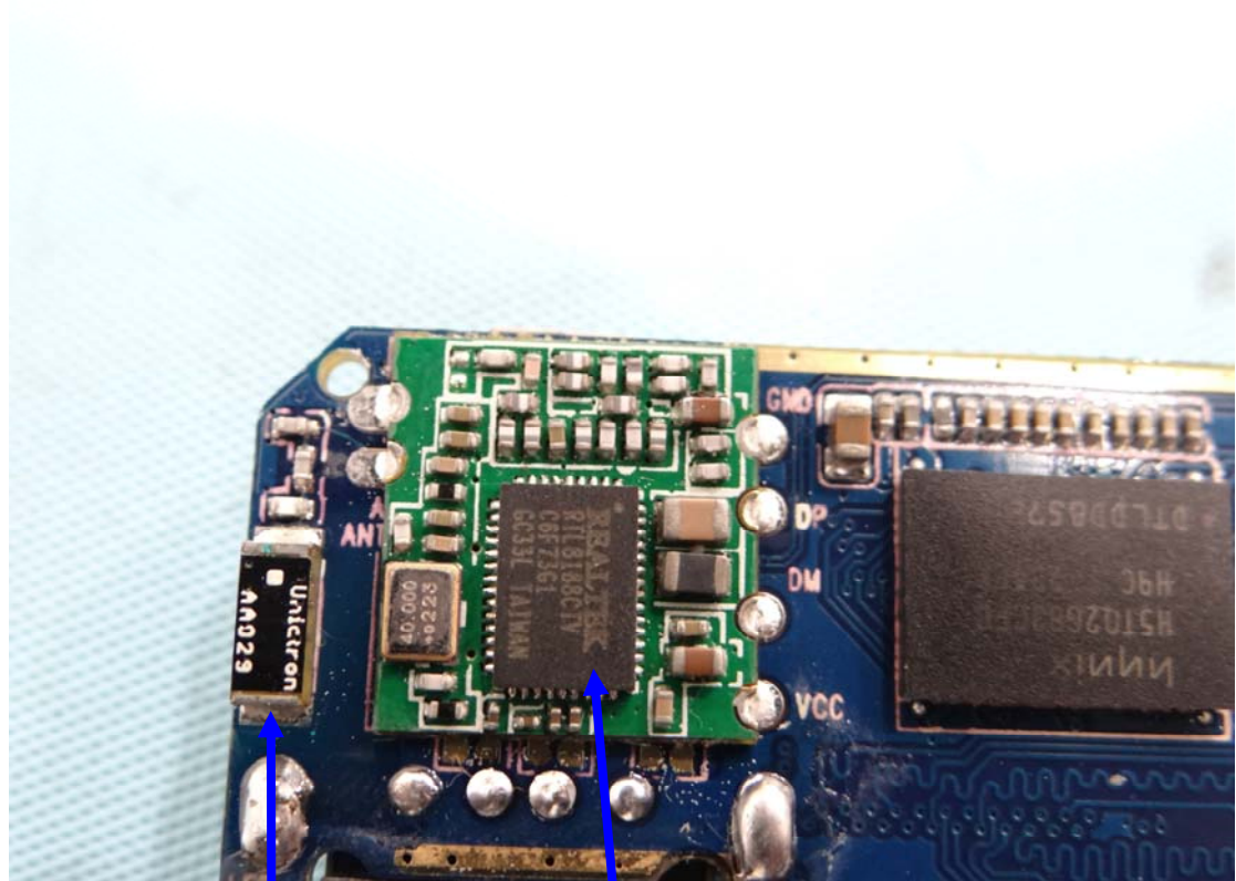
Antenna
