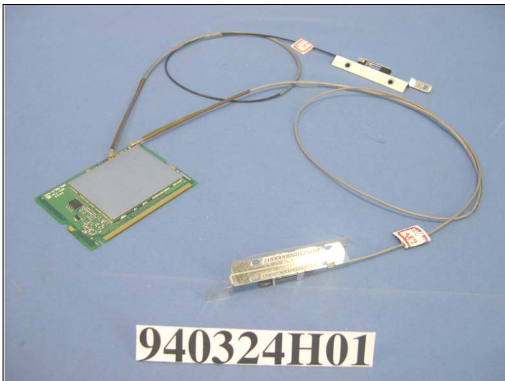
Antenna 1, 2
