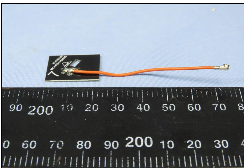
5GH/6E ANT 3
