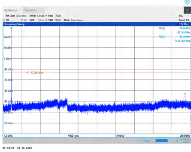
Band25-20MHz-QPSK-26140-1RB#0-Range4:1000~20000MHz
