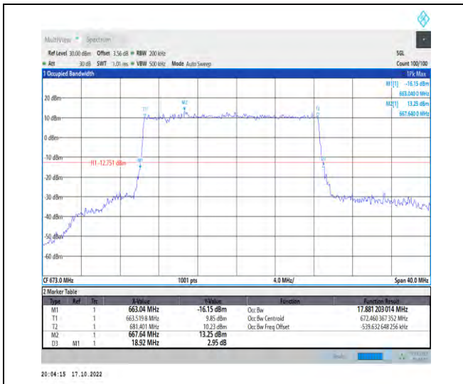
1-N71-PC3-15-20-L-1-DFT-QPSK-Outer_Full-100@ 0-Ant1-17.881-18.920-≤20-PASS
