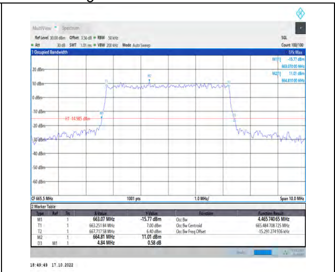
1-N71-PC3-15-5-L-7-CP-16QAM-Outer_Full-25@0-A Ant1-4.466-4.840-≤5-PASS
