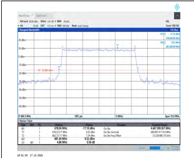
1-N71-PC3-15-5-M-6-CP-QPSK-Outer_Full-25@0-A nt1-4.467-4.860-<math>\leq</math>5-PASS
