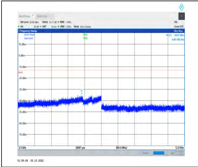
1-N66-PC3-15-40-L-1-DFT-QPSK-Inner_1RB_Left-1 @1-3000-12000-Ant1-6451.05--34.57--13-PASS
