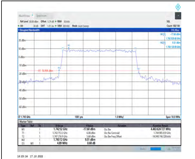
1-N66-PC3-15-5-M-6-CP-QPSK-Outer_Full-25@0-A nt1-4.464-4.890-<math>\leq</math>5-PASS
