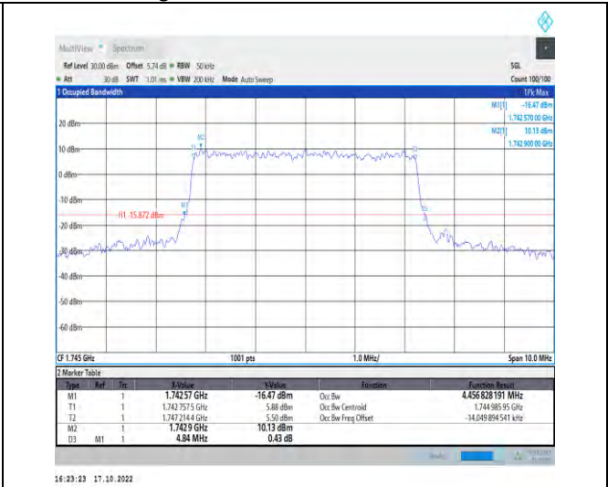
1-N66-PC3-15-5-M-7-CP-16QAM-Outer_Full-25@0-A nt1-4.457-4.840-<math>\leq</math>5-PASS
