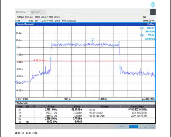
1-N41-PC2-30-70-L-9-CP-256QAM-Outer_Full-189@0 0-Ant1-67.406-69.720-≤70-PASS
