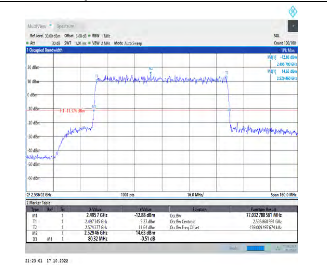
1-N41-PC2-30-80-L-3-DFT-16QAM-Outer_Full-216@ 0-Ant1-77.033-80.320-≤80-PASS
