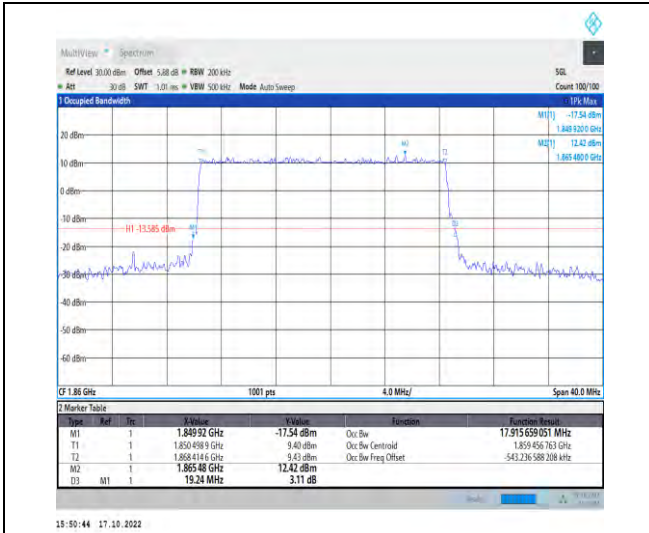
1-N25-PC3-15-20-L-1-DFT-QPSK-Outer_Full-100@ 0-Ant1-17.916-19.240-≤20-PASS
