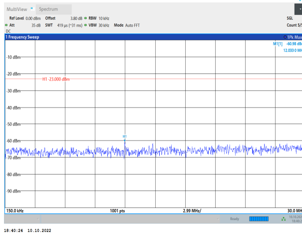
Band71-20MHz-QPSK-133222-1RB#0-Range2:0.15~30MHz
