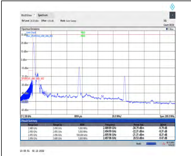
1-41-41-30-80+40-L-1-DFT-QPSK-Edge_1RB_Left
