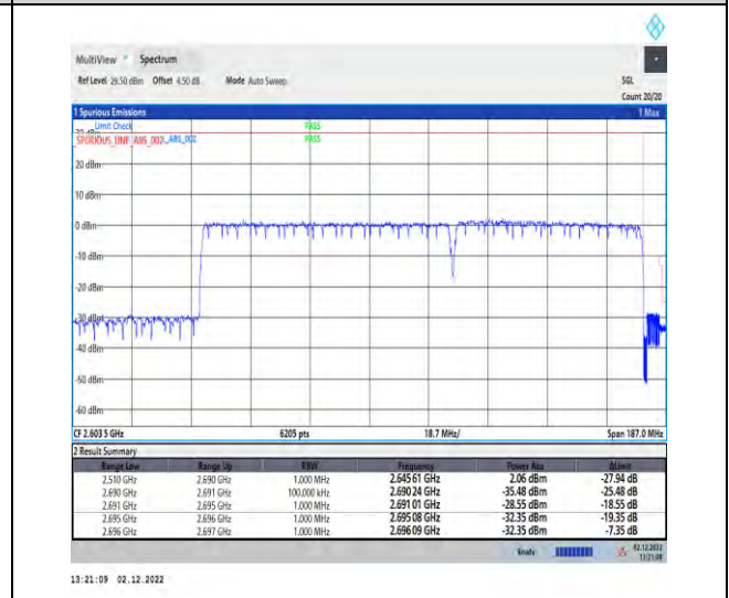
1-41-41-30-80+60-H-3-DFT-QPSK-Outer_Full
