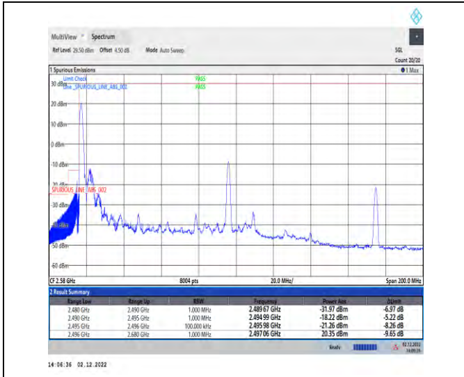
1-41-41-30-100+60-L-5-CP-QPSK-Edge_1RB_Left
