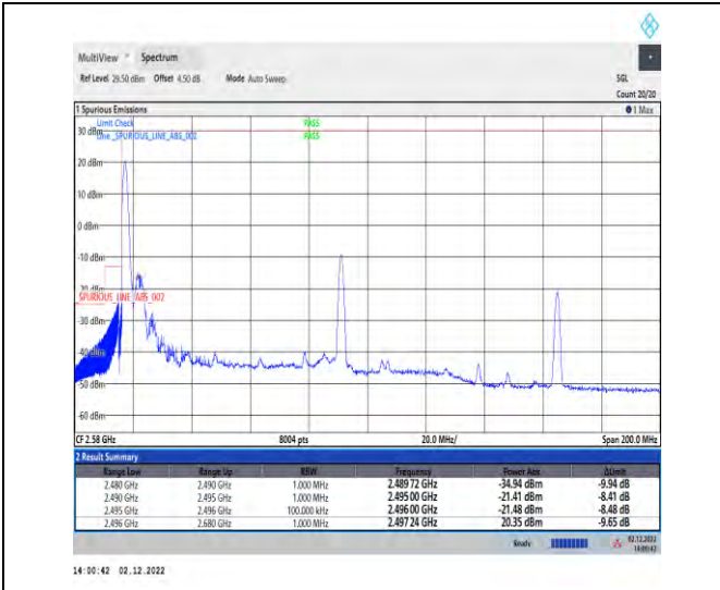
1-41-41-30-80+80-L-4-CP-QPSK-Edge_1RB_Left
