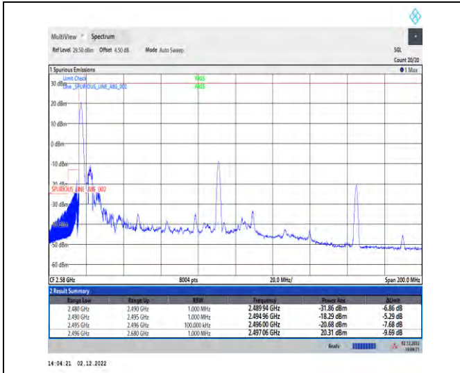
1-41-41-30-100+50-L-4-CP-QPSK-Edge_1RB_Left
