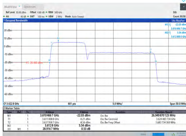
48-48-10MHz-20MHz-QPSK-QPSK-55896-56040-50RB#0-100RB#0
