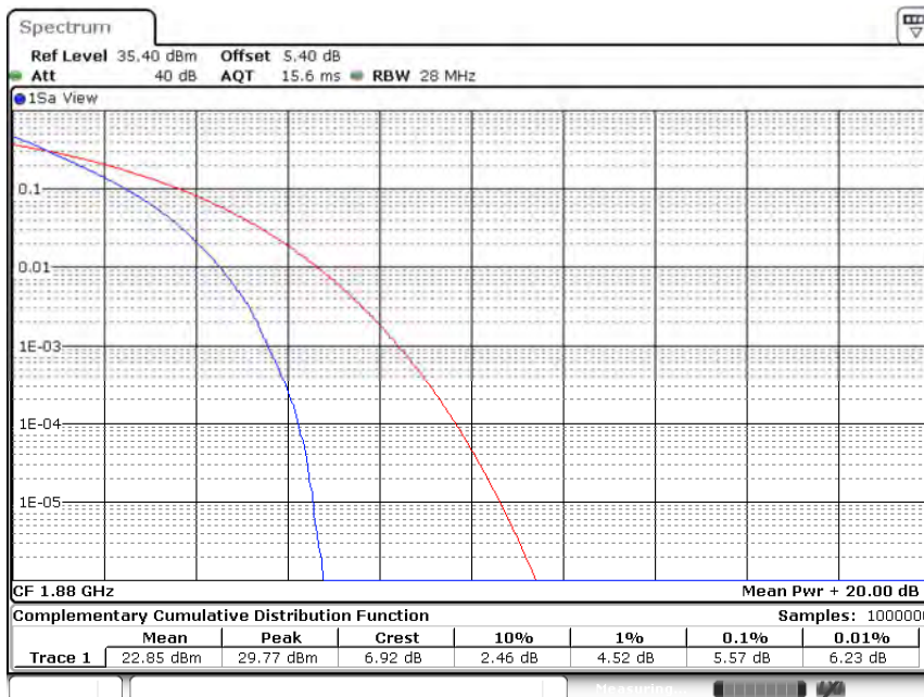
Band2-20MHz-QPSK-18900-100RB#0
