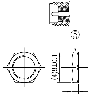
NUT
