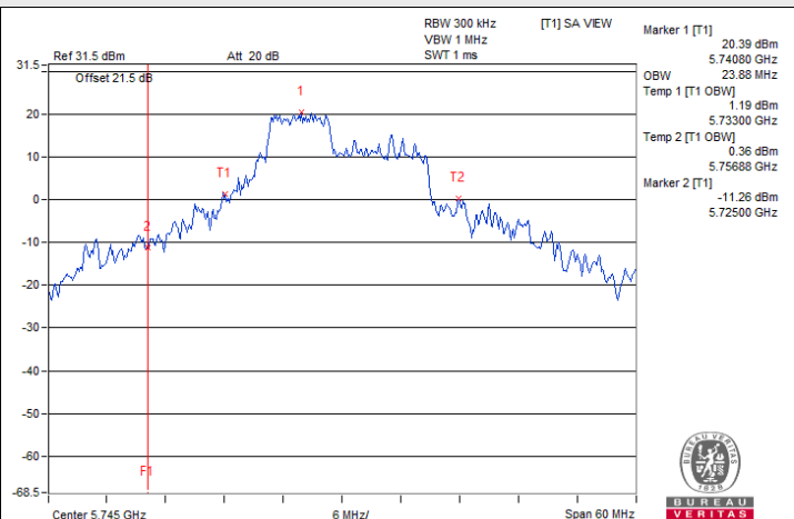
802.11be (EHT20) 52+26-tone MRU / Chain 0 : CH 149@70 802.11be (EHT20) 52+26-tone MRU / Chain 1 : CH 149@70
