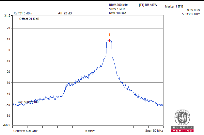
802.11be (EHT) 26-tone RU / Chain 0 : CH 165@8
