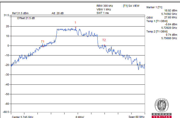
802.11be (EHT20) 106+26-tone MRU / Chain 1 : CH 149@82
