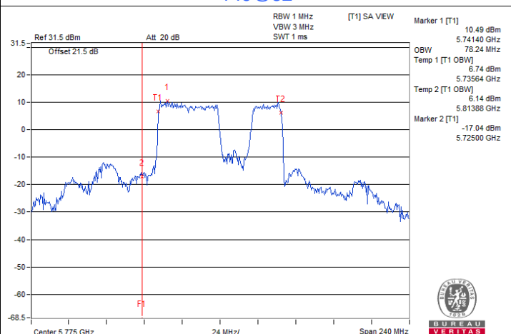
802.11be (EHT80) 484+242-tone MRU / Chain 1 : CH 155@92
