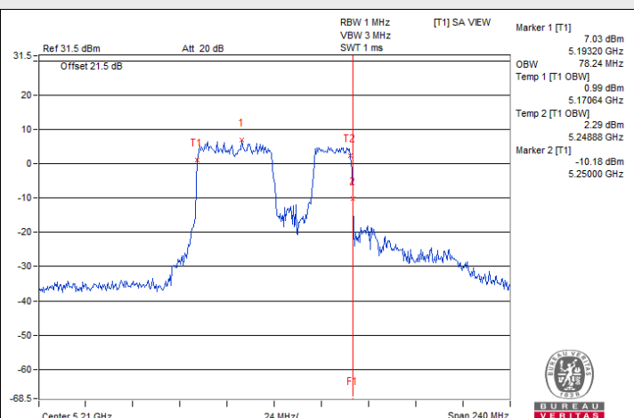
802.11be (EHT80) 484+242-tone MRU / Chain 1 : CH 42@92
