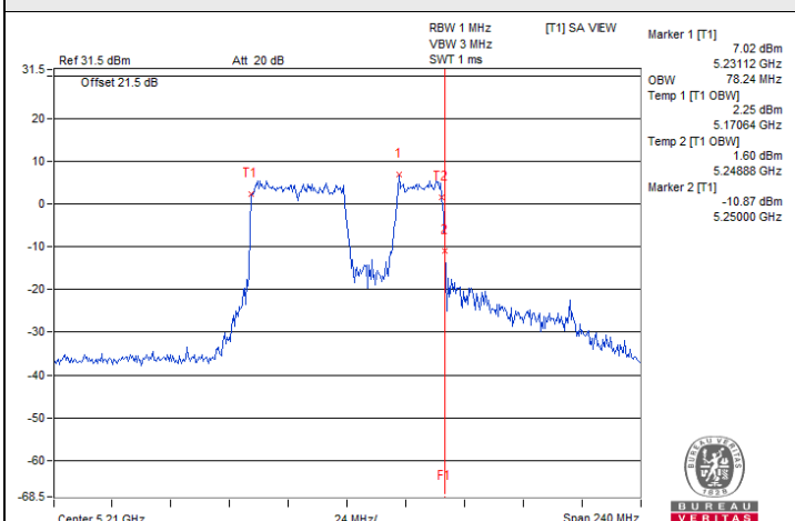
802.11be (EHT80) 484+242-tone MRU / Chain 0 : CH 42@92
