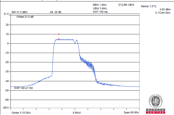
802.11be (EHT20) 106+26-tone MRU / Chain 0 : CH 36@82
