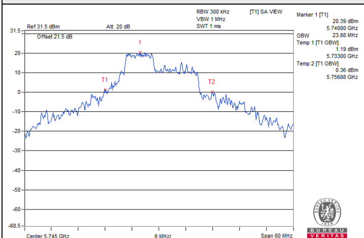
802.11be (EHT20) 52+26-tone MRU / Chain 1 : CH 149@70
