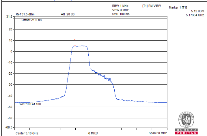
802.11be (EHT20) 52+26-tone MRU / Chain 1 : CH 36@70
