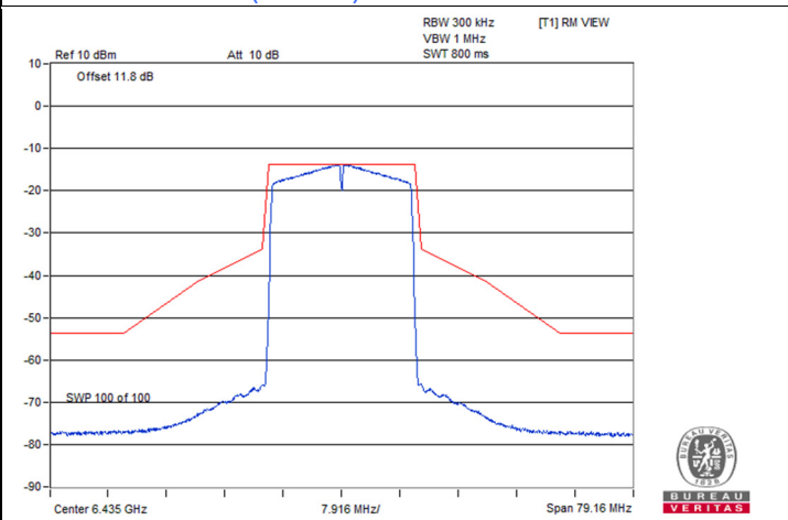
802.11be (EHT20) 2S2T / Chain 1 : CH 97
