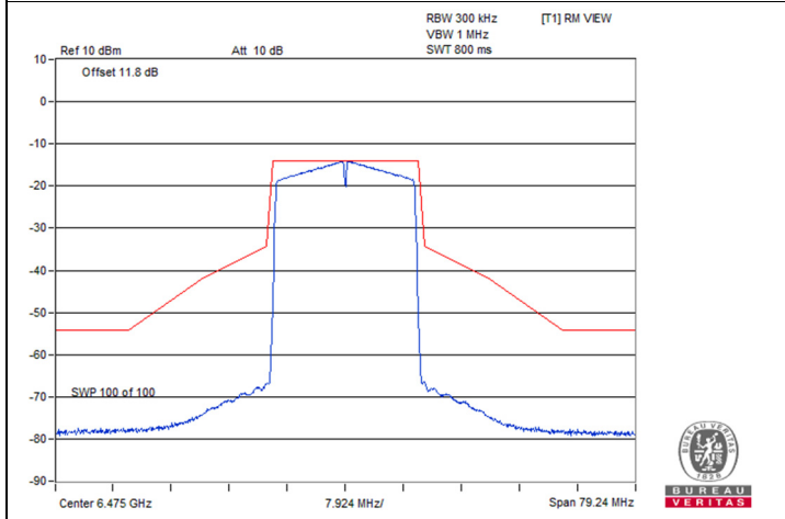
802.11be (EHT20) 2S2T / Chain 1 : CH 105
