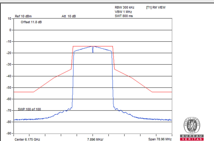
802.11be (EHT20) 2S2T / Chain 1 : CH 45
