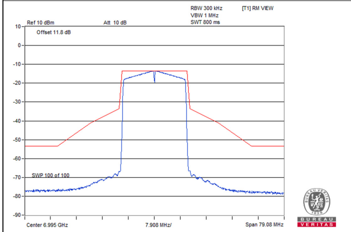
802.11be (EHT20) 2S2T / Chain 1 : CH 209
