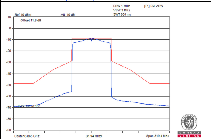
802.11be (EHT80) 2S2T / Chain 1 : CH 183
