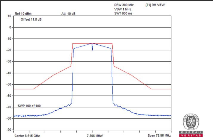
802.11be (EHT20) 2S2T / Chain 1 : CH 113
