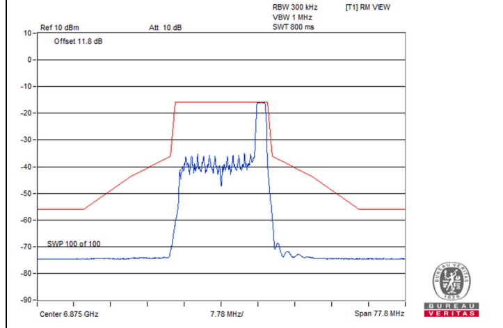
802.11be (EHT20) 26-tone RU 2S2T / Chain 0 : CH 185
