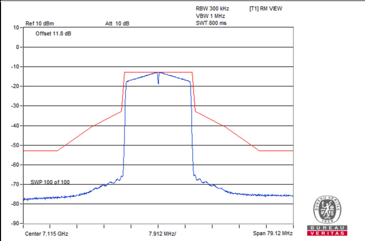
802.11be (EHT20) 2S2T / Chain 1 : CH 233
