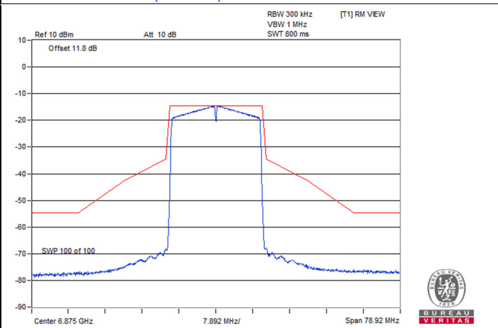
802.11be (EHT20) 2S2T / Chain 1 : CH 185
