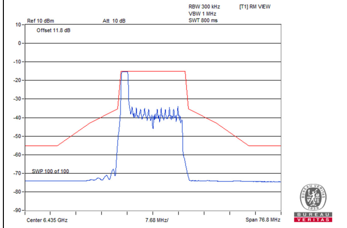
802.11be (EHT20) 26-tone RU 2S2T / Chain 0 : CH 97
