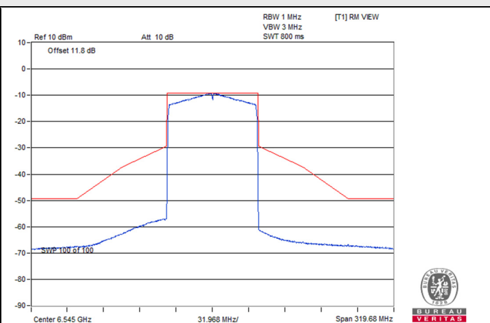
802.11be (EHT80) 2S2T / Chain 1 : CH 119
