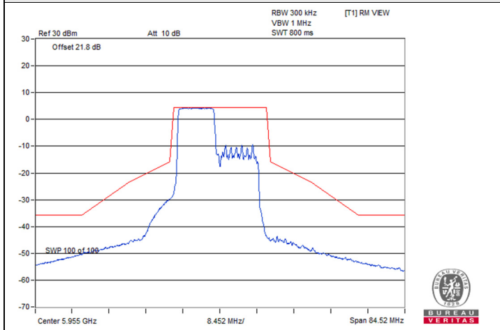
802.11be (EHT20) 106-tone RU 2S2T / Chain 0 : CH 1
