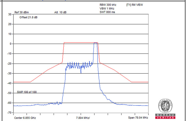
802.11be (EHT20) 26-tone RU 2S2T / Chain 0 : CH 181
