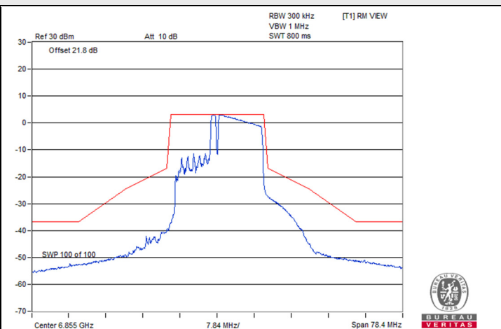
802.11be (EHT20) 106+26-tone MRU 2S2T / Chain 1 : CH 181
