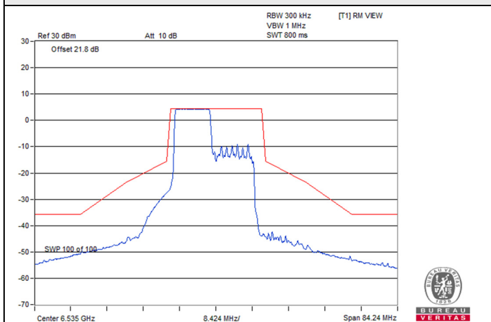
802.11be (EHT20) 106-tone RU 2S2T / Chain 1 : CH 117
