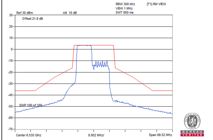
802.11be (EHT20) 106-tone RU 2S2T / Chain 0 : CH 117
