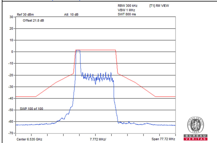
802.11be (EHT20) 26-tone RU 2S2T / Chain 0 : CH 117
