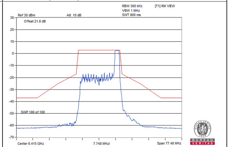
802.11be (EHT20) 26-tone RU 2S2T / Chain 1 : CH 93
