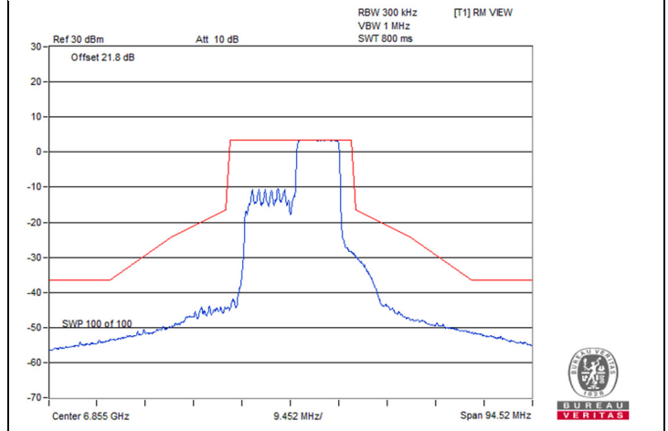
802.11be (EHT20) 106-tone RU 2S2T / Chain 0 : CH 181
