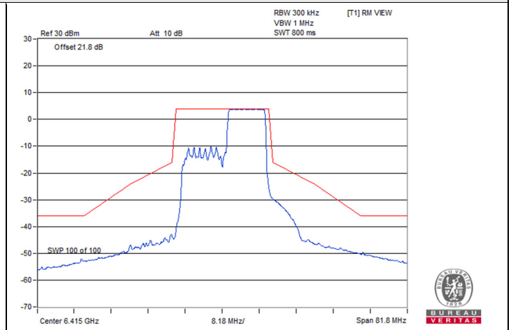
802.11be (EHT20) 106-tone RU 2S2T / Chain 0 : CH 93
