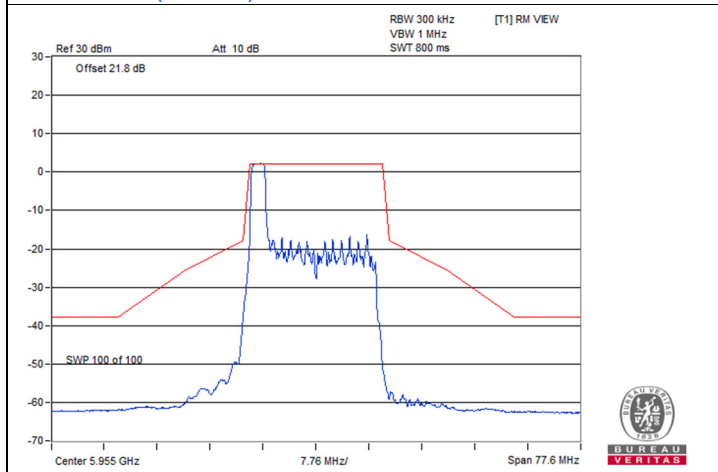
802.11be (EHT20) 26-tone RU 2S2T / Chain 1 : CH 1
