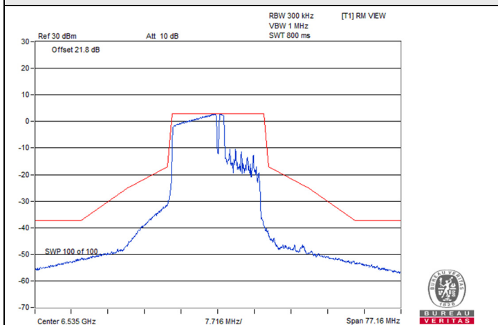
802.11be (EHT20) 106+26-tone MRU 2S2T / Chain 1 : CH 117
