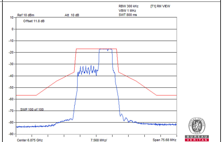
802.11be (EHT20) 52+26-tone MRU 2S2T / Chain 0 : CH 185
