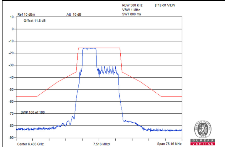
802.11be (EHT20) 52+26-tone MRU 2S2T / Chain 0 : CH 97
