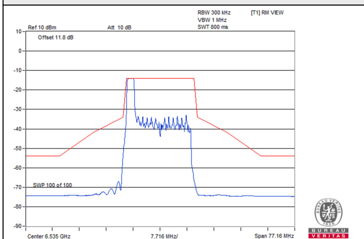
802.11be (EHT20) 26-tone RU 2S2T / Chain 1 : CH 117
