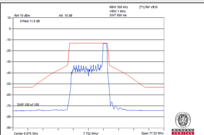
802.11be (EHT20) 26-tone RU 2S2T / Chain 1 : CH 185
