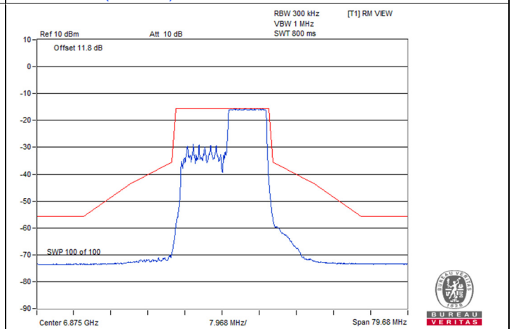
802.11be (EHT20) 106-tone RU 2S2T / Chain 0 : CH 185
