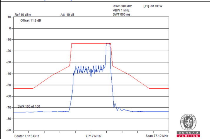
802.11be (EHT20) 26-tone RU 2S2T / Chain 1 : CH 233
