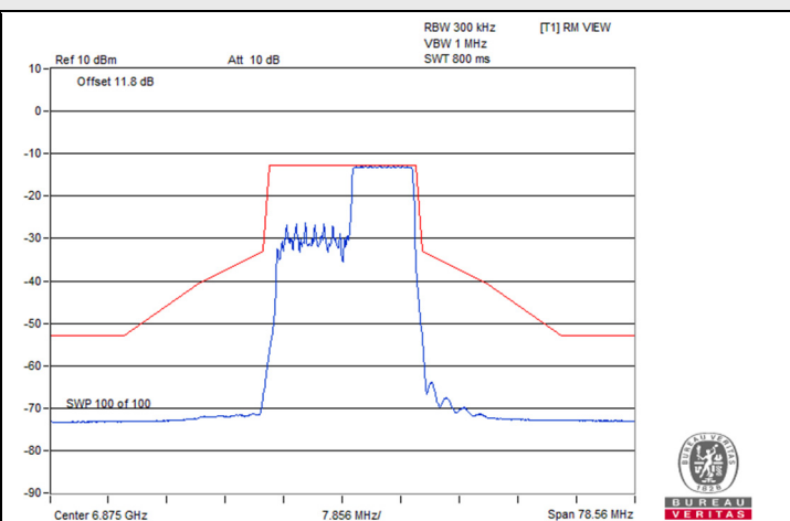
802.11be (EHT20) 106-tone RU 2S2T / Chain 1 : CH 185
