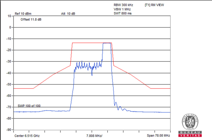
802.11be (EHT20) 52-tone RU 2S2T / Chain 1 : CH 113
