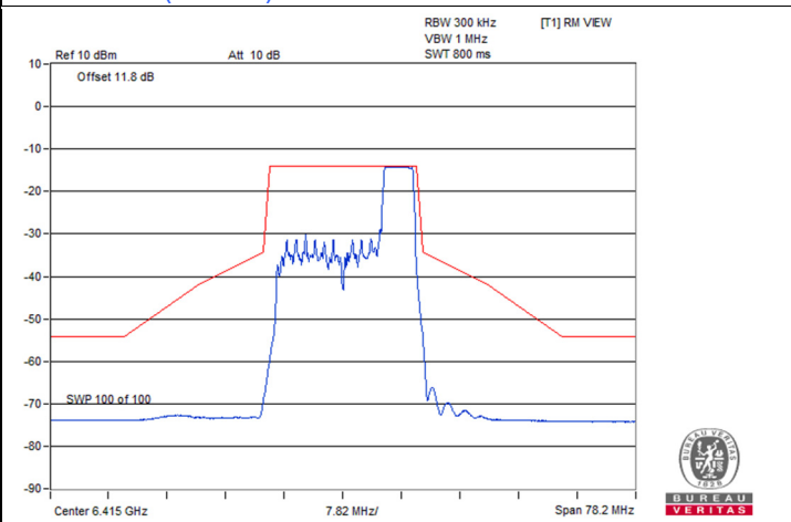
802.11be (EHT20) 52-tone RU 2S2T / Chain 1 : CH 93
