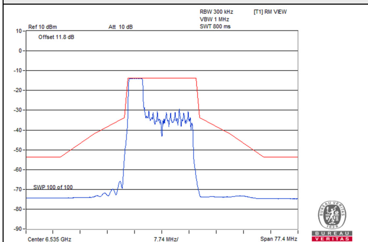
802.11be (EHT20) 52-tone RU 2S2T / Chain 1 : CH 117
