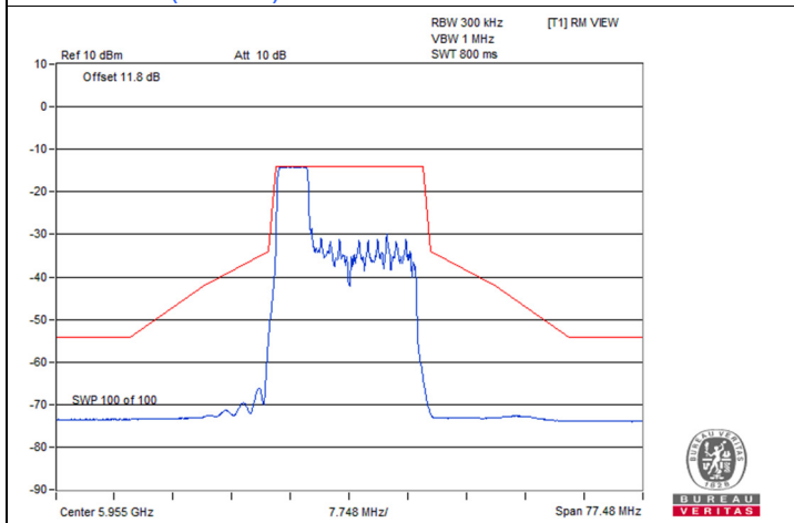
802.11be (EHT20) 52-tone RU 2S2T / Chain 1 : CH 1
