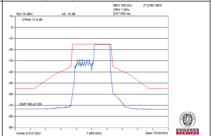
802.11be (EHT20) 106-tone RU 2S2T / Chain 0 : CH 113
