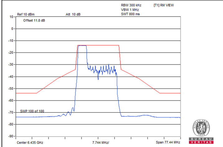
802.11be (EHT20) 52-tone RU 2S2T / Chain 1 : CH 97
