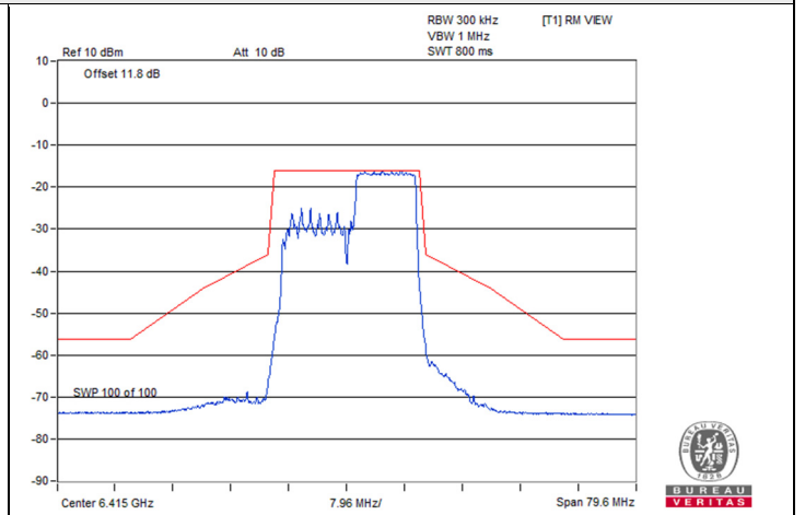
802.11be (EHT20) 106-tone RU 2S2T / Chain 0 : CH 93
