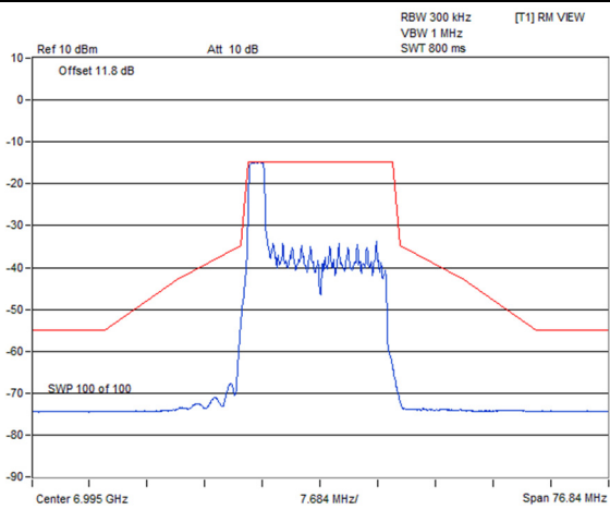
802.11be (EHT20) 26-tone RU 2S2T / Chain 0 : CH 209
