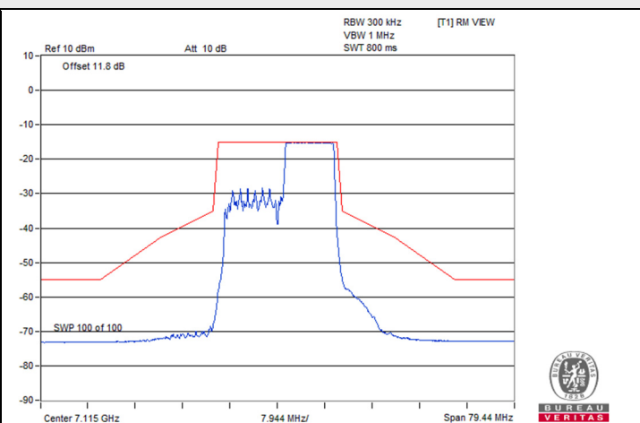
802.11be (EHT20) 106-tone RU 2S2T / Chain 0 : CH 233
