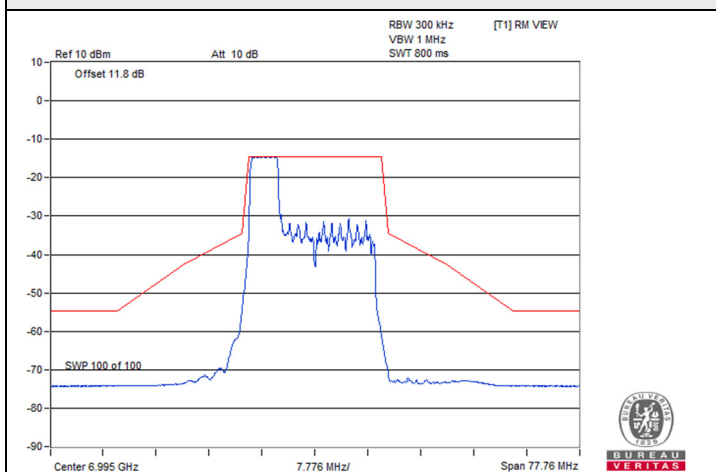
802.11be (EHT20) 52-tone RU 2S2T / Chain 0 : CH 209
