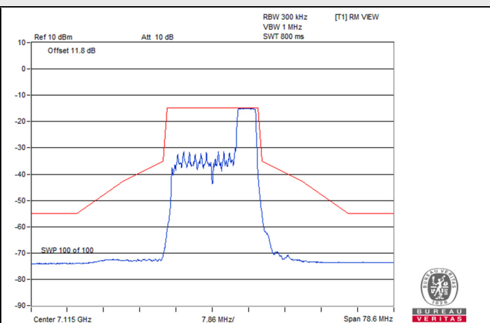
802.11be (EHT20) 52-tone RU 2S2T / Chain 0 : CH 233
