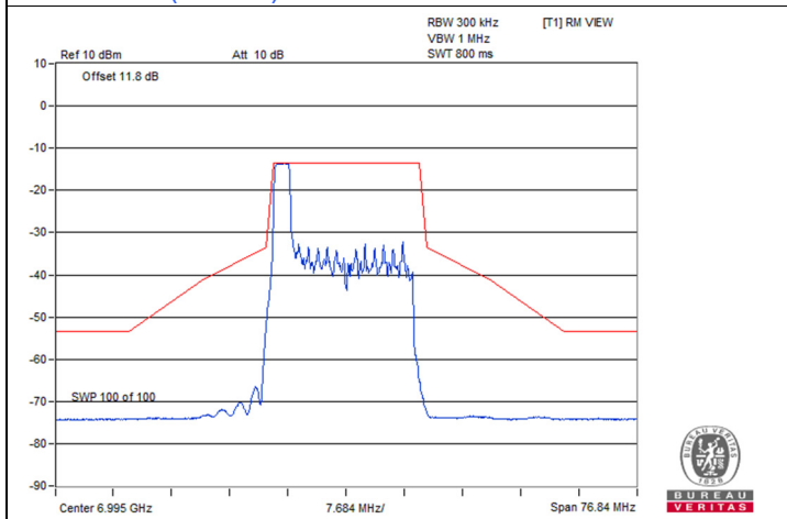
802.11be (EHT20) 26-tone RU 2S2T / Chain 1 : CH 209
