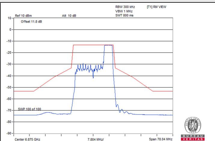
802.11be (EHT20) 52-tone RU 2S2T / Chain 1 : CH 185
