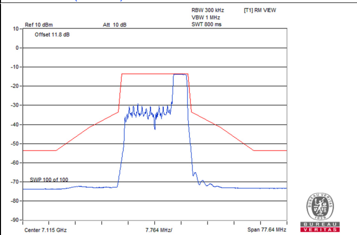
802.11be (EHT20) 52-tone RU 2S2T / Chain 1 : CH 233
