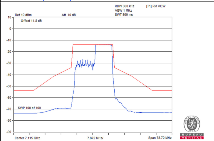
802.11be (EHT20) 106-tone RU 2S2T / Chain 1 : CH 233
