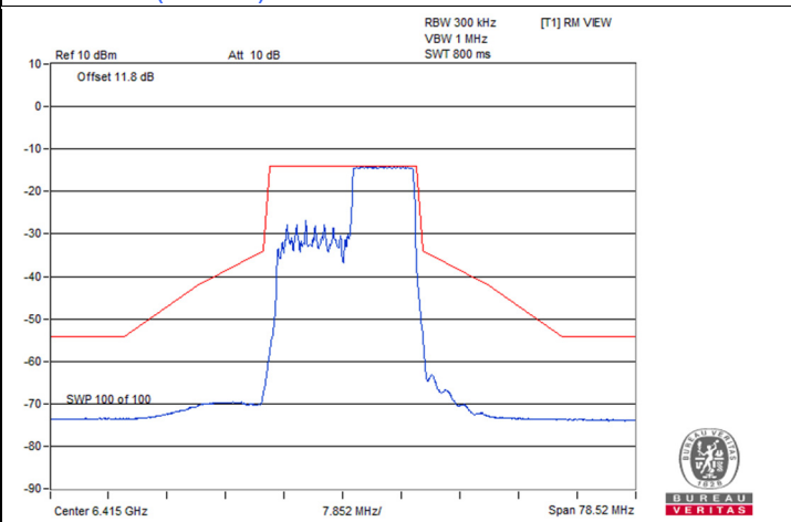
802.11be (EHT20) 106-tone RU 2S2T / Chain 1 : CH 93
