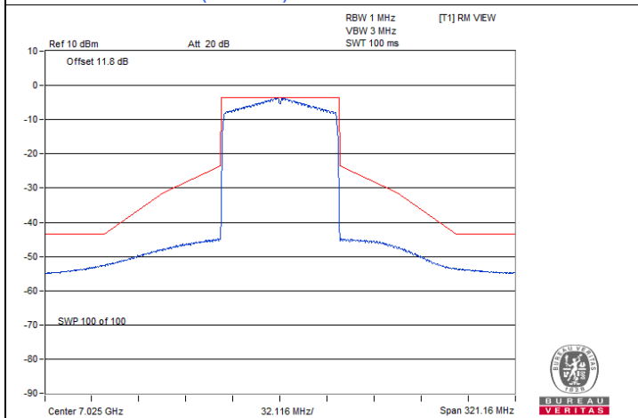
802.11be (EHT80) 1S1T / Chain 0 : CH 215
