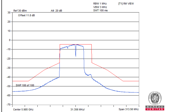
802.11be (EHT80) 484+242-tone MRU 1S1T / Chain 0 : CH 7
