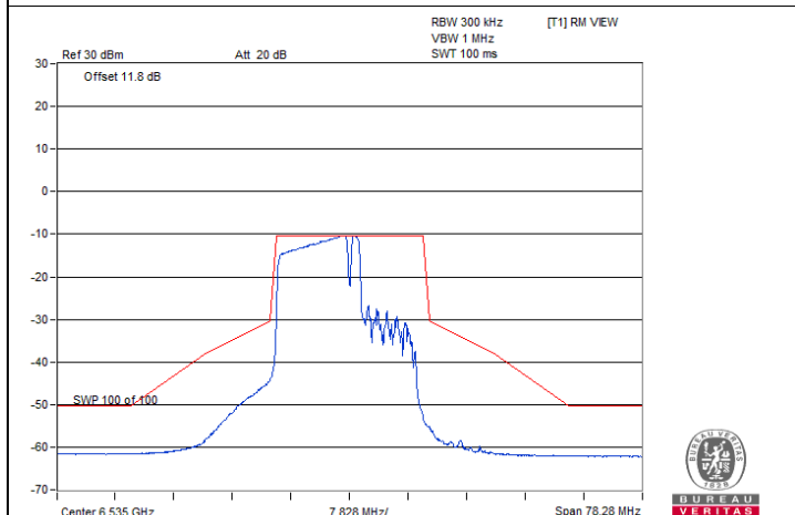
802.11be (EHT20) 106+26-tone MRU 1S1T / Chain 0 : CH 117
