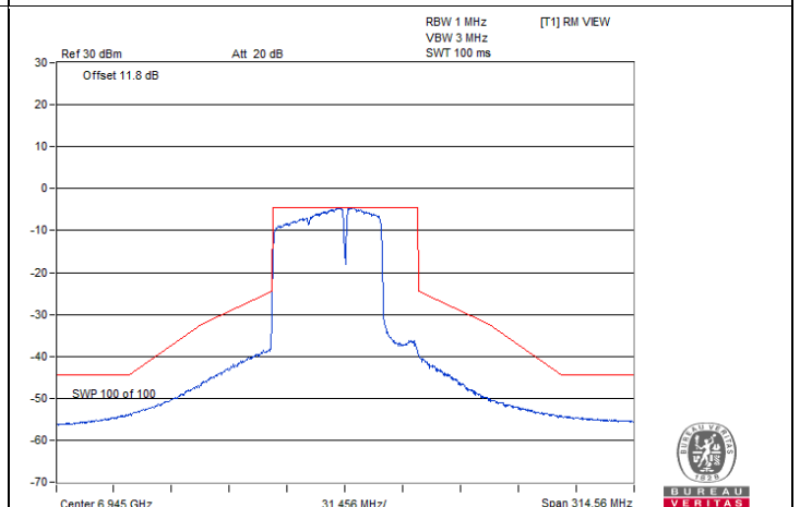
802.11be (EHT80) 484+242-tone MRU 1S1T / Chain 0 : CH 199
