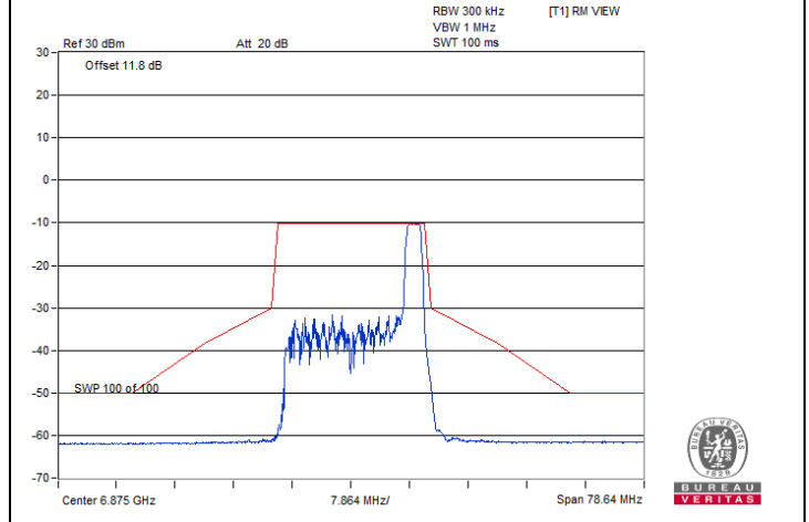
802.11be (EHT20) 26-tone RU 1S1T / Chain 0 : CH 185
