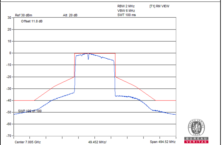
802.11be (EHT160) 996+484-tone MRU 1S1T / Chain 0 : CH 207
