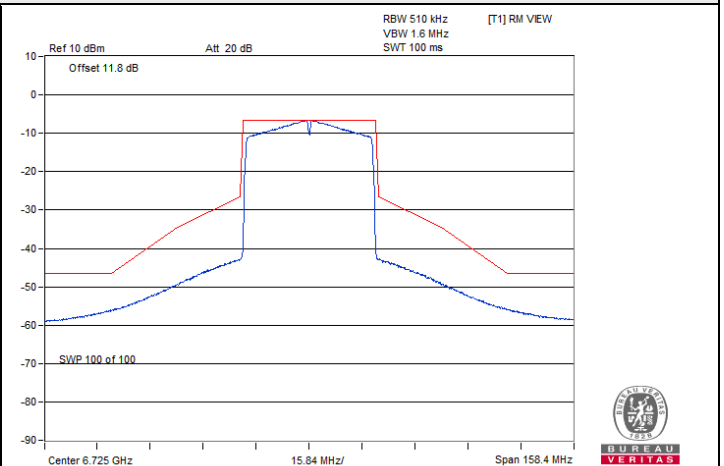
802.11be (EHT40) 1S1T / Chain 0 : CH 155
