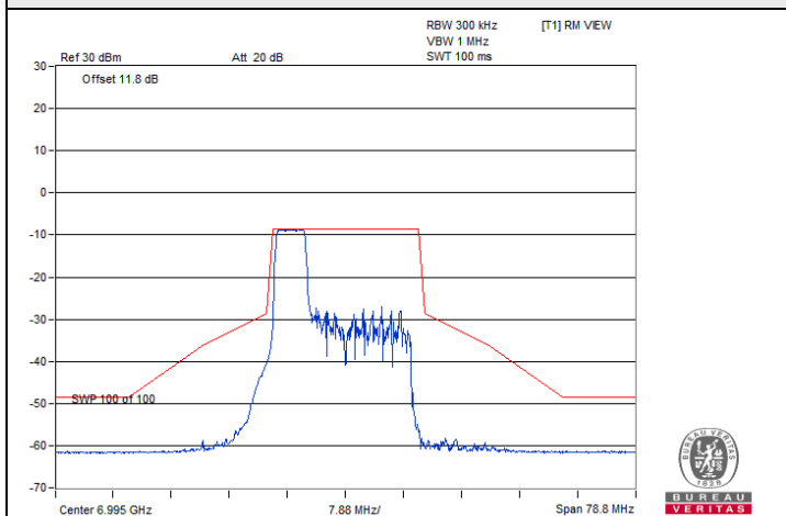
802.11be (EHT20) 52-tone RU 1S1T / Chain 0 : CH 209
