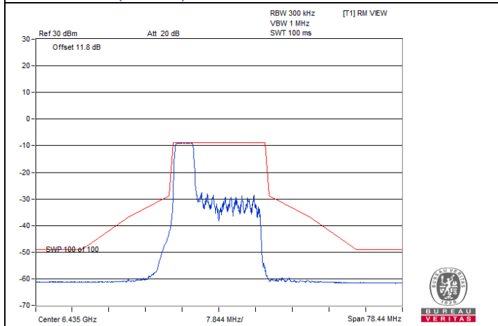
802.11be (EHT20) 52-tone RU 1S1T / Chain 0 : CH 97
