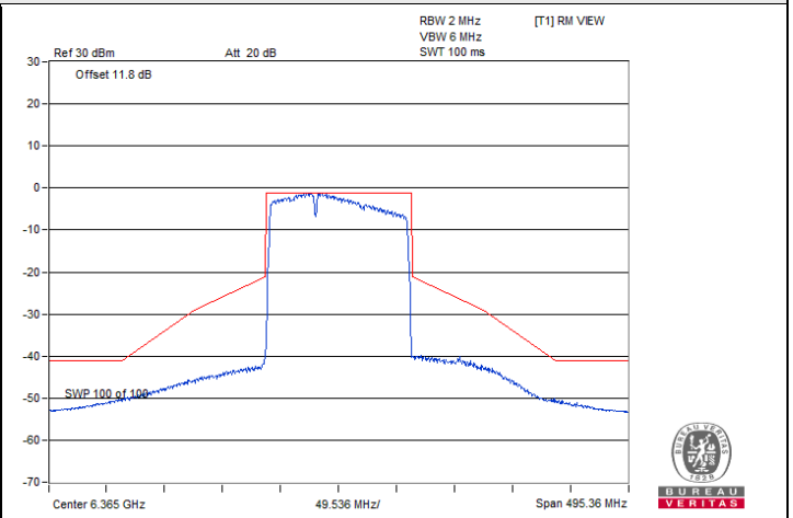
802.11be (EHT160) 996+484-tone MRU 1S1T / Chain 0 : CH 79
