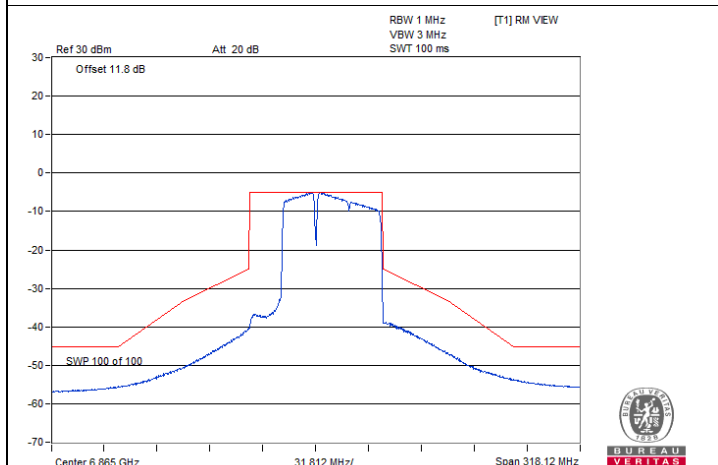
802.11be (EHT80) 484+242-tone MRU 1S1T / Chain 0 : CH 183
