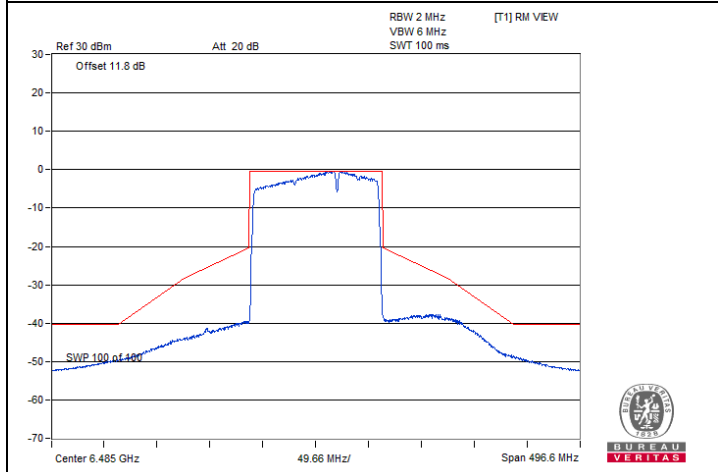
802.11be (EHT160) 996+484-tone MRU 1S1T / Chain 0 : CH 111
