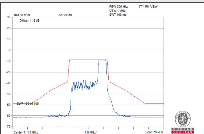
802.11be (EHT20) 52-tone RU 1S1T / Chain 0 : CH 233
