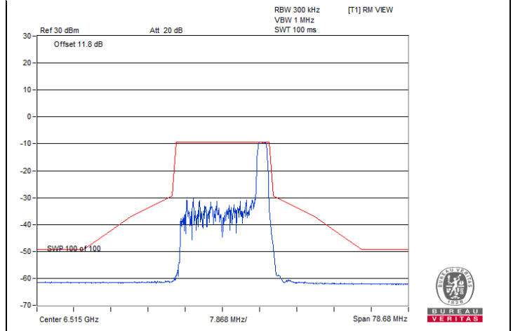
802.11be (EHT20) 26-tone RU 1S1T / Chain 0 : CH 113
