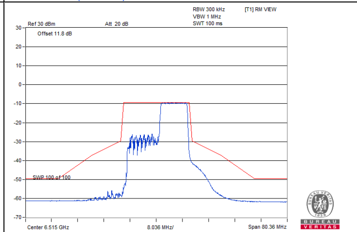
802.11be (EHT20) 106-tone RU 1S1T / Chain 0 : CH 113
