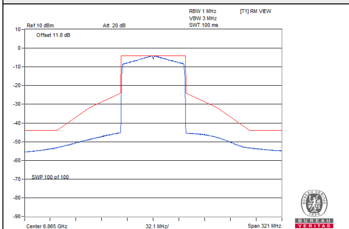
802.11be (EHT80) 1S1T / Chain 0 : CH 183
