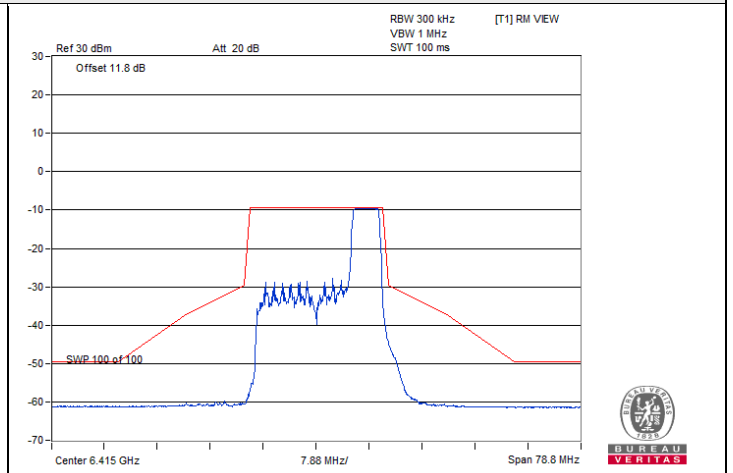
802.11be (EHT20) 52-tone RU 1S1T / Chain 0 : CH 93
