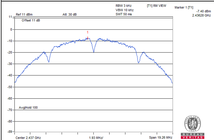
802.11b 1TX / Chain 0 : CH 6
