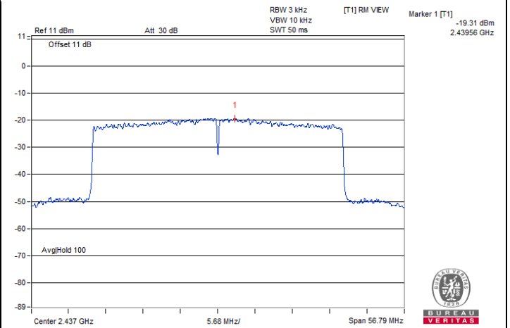
802.11be (EHT40) 1S1T / Chain 0 : CH 6
