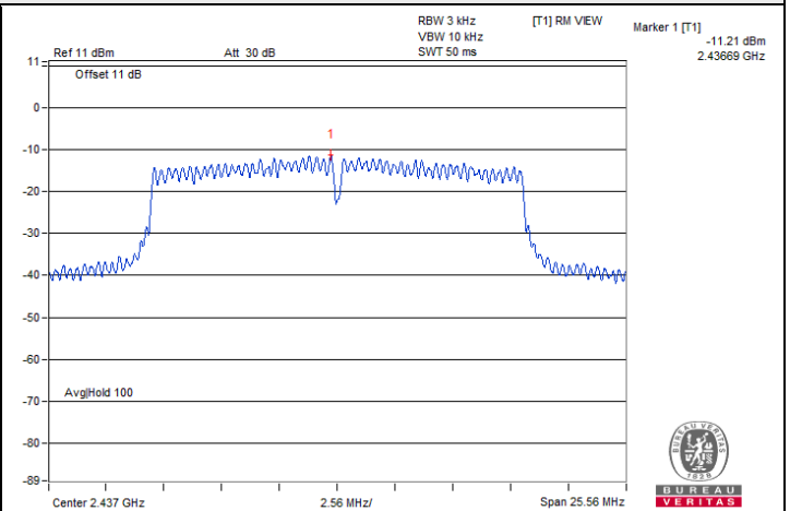
802.11g 1TX / Chain 0 : CH 6
