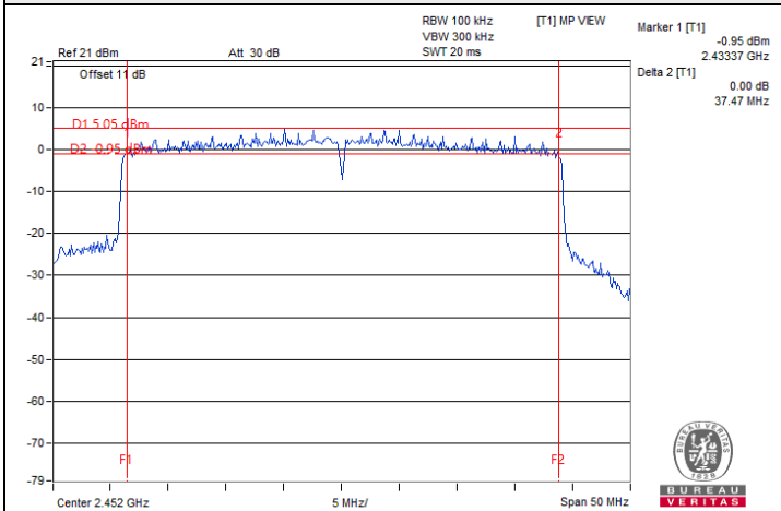
802.11be (EHT40) 2S2T / Chain 0 : CH 9
