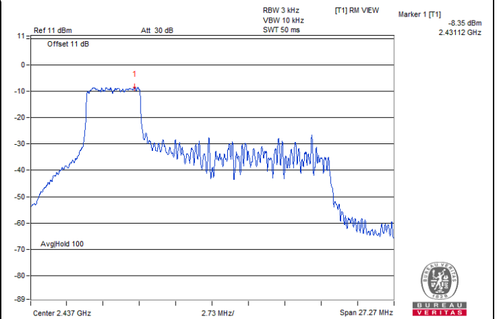
802.11be (EHT20) 52-tone RU 1S1T / Chain 0 : CH 6@37
