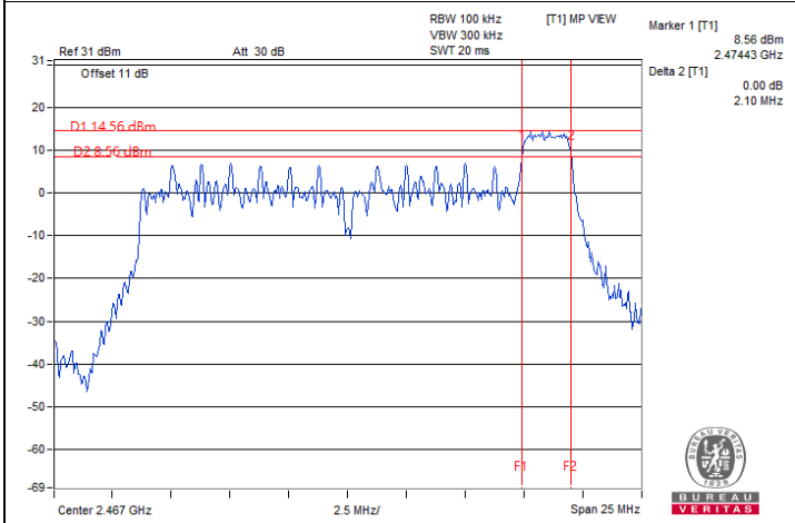
802.11be (EHT20) 26-tone RU 1S1T / Chain 0 : CH 12@8
