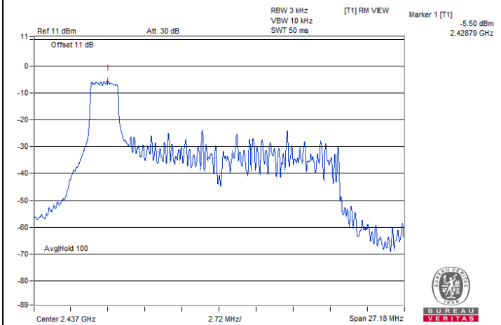
802.11be (EHT20) 26-tone RU 1S1T / Chain 0 : CH 6@0
