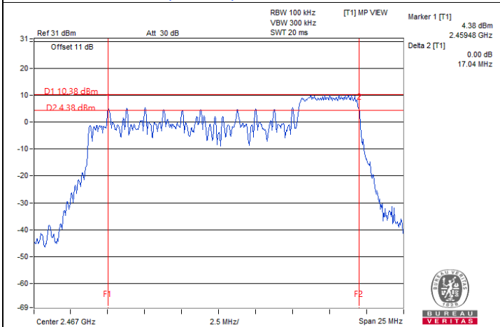
802.11be (EHT20) 52-tone RU 2S2T / Chain 0 : CH 12@40
