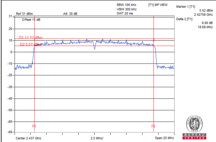
802.11be (EHT20) 1S1T / Chain 0 : CH 6
