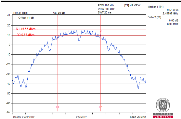
802.11b 1TX / Chain 0 : CH 11
