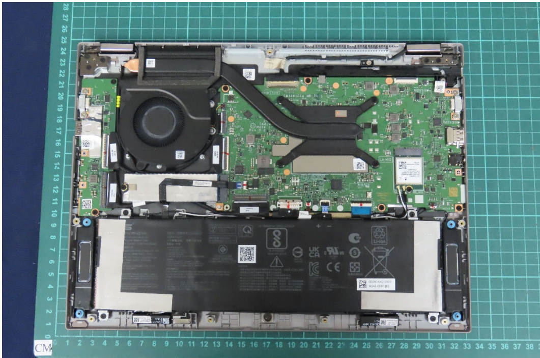
(15) EUT Photo
