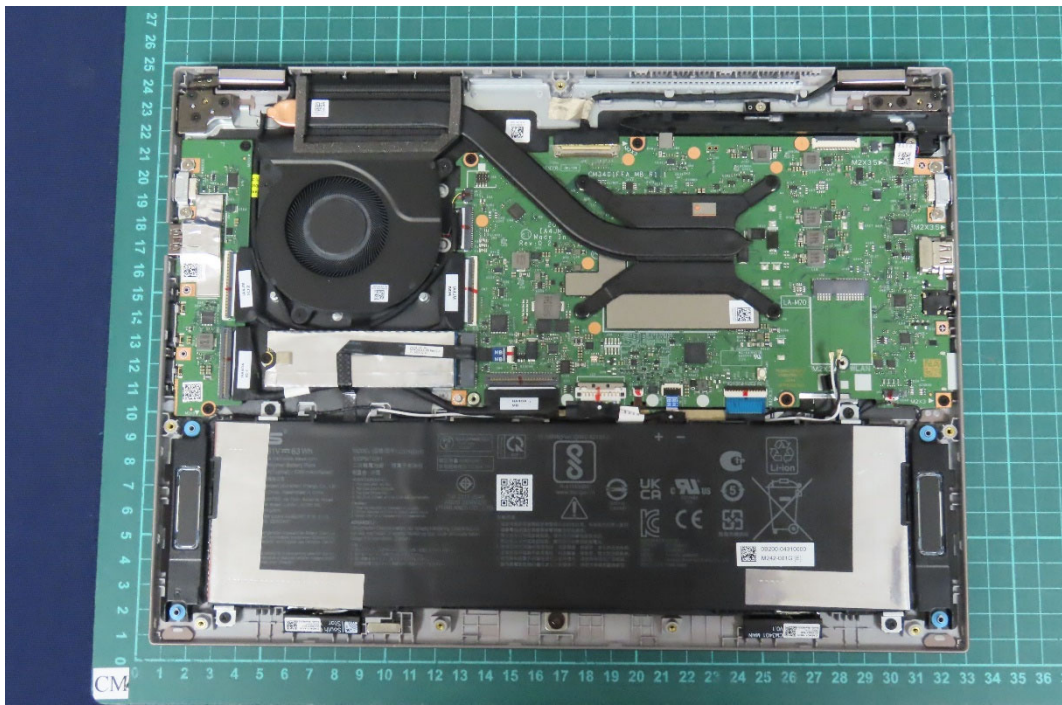
(19) EUT Photo
