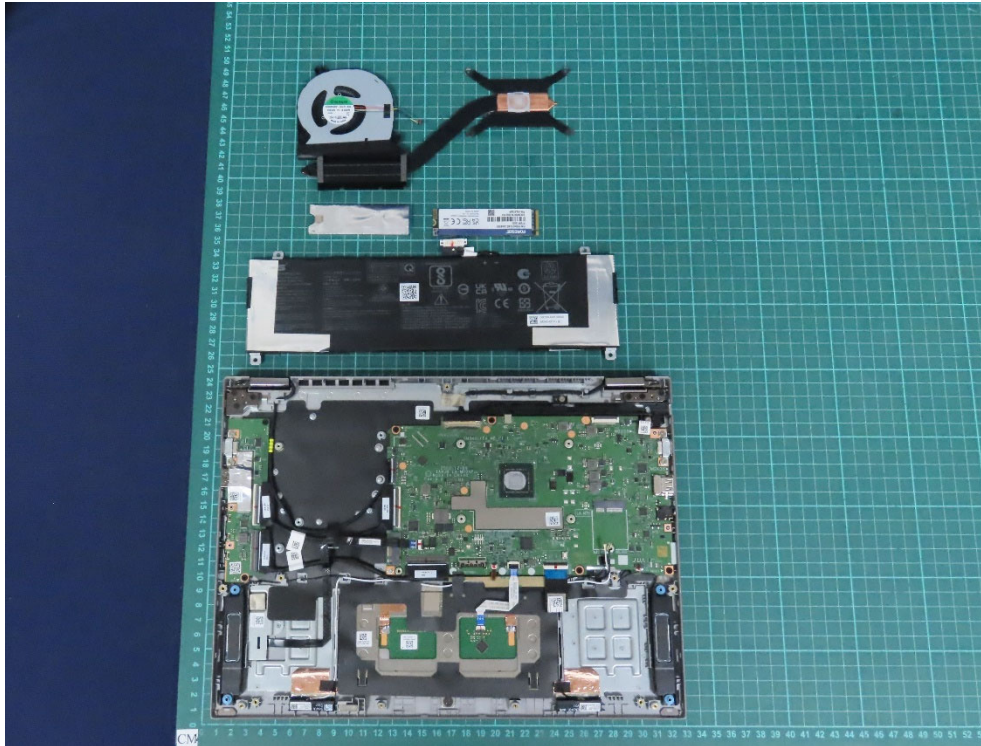
(20) EUT Photo
