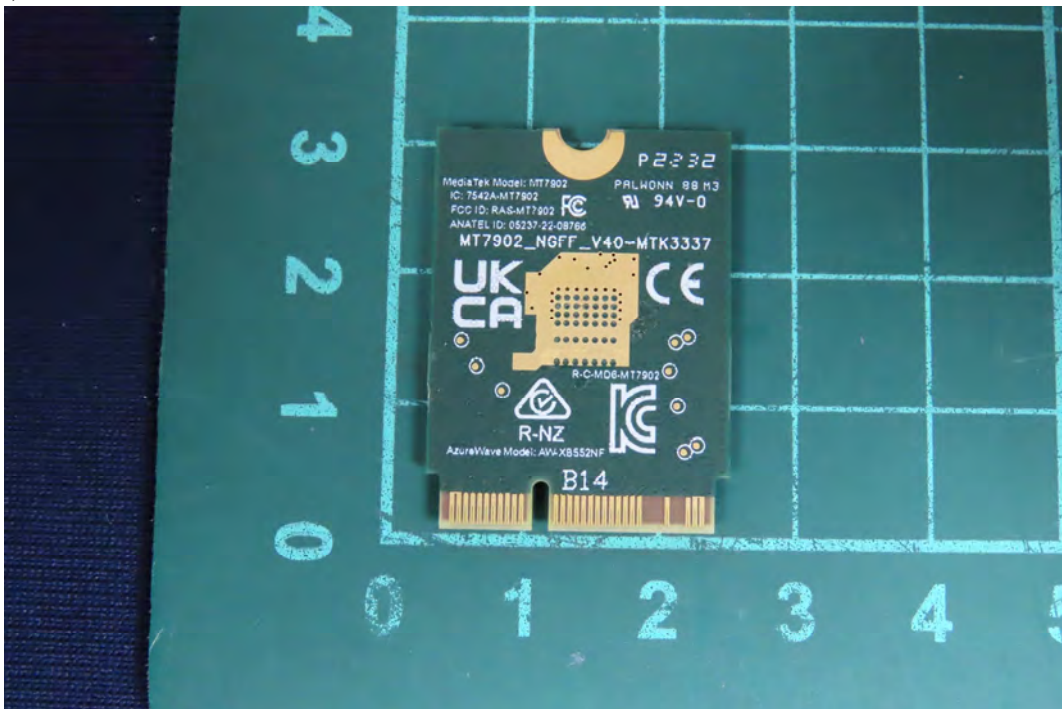
(6) EUT Photo_MT7902
