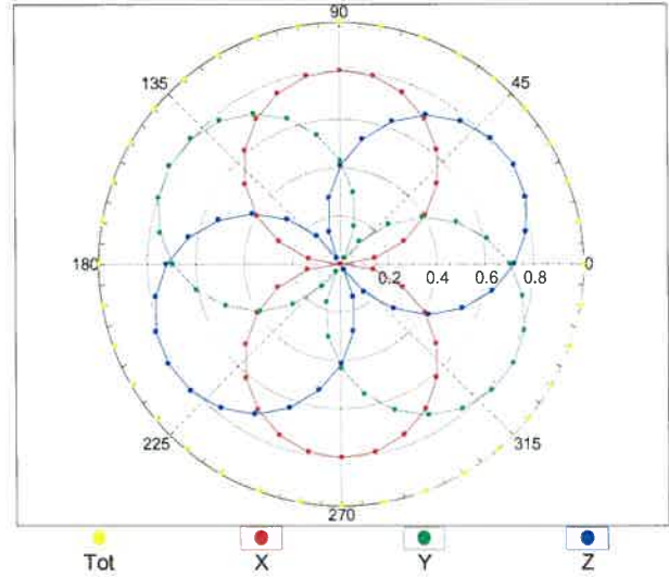
f=1800 MHz,R22
