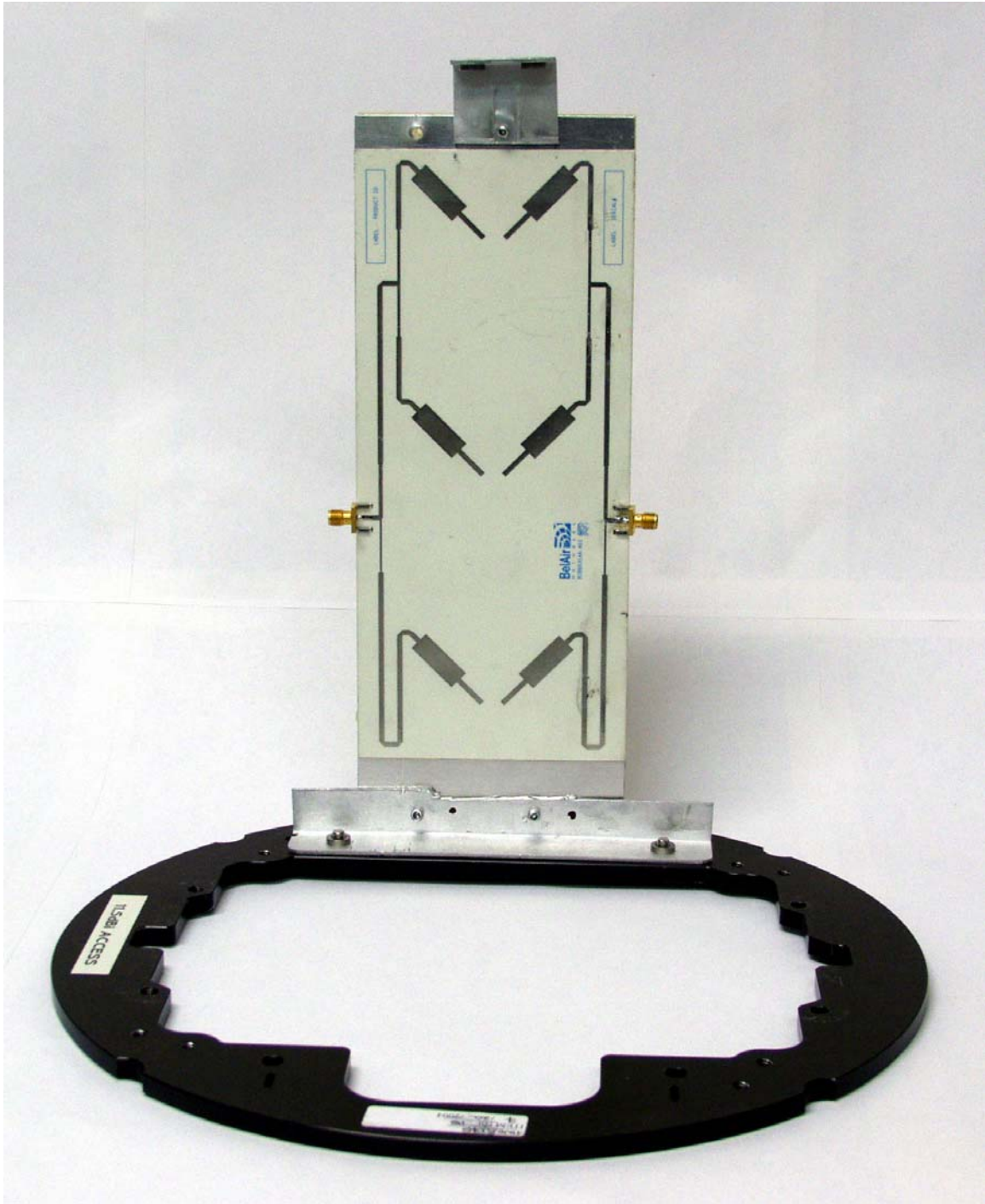
12dBi Antenna_BelAir_rear
