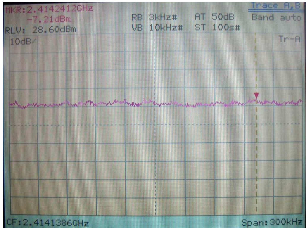
IEEE 802.11b
