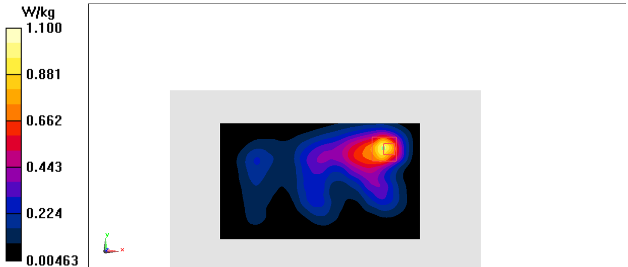
Fig.14 LTE Band7
