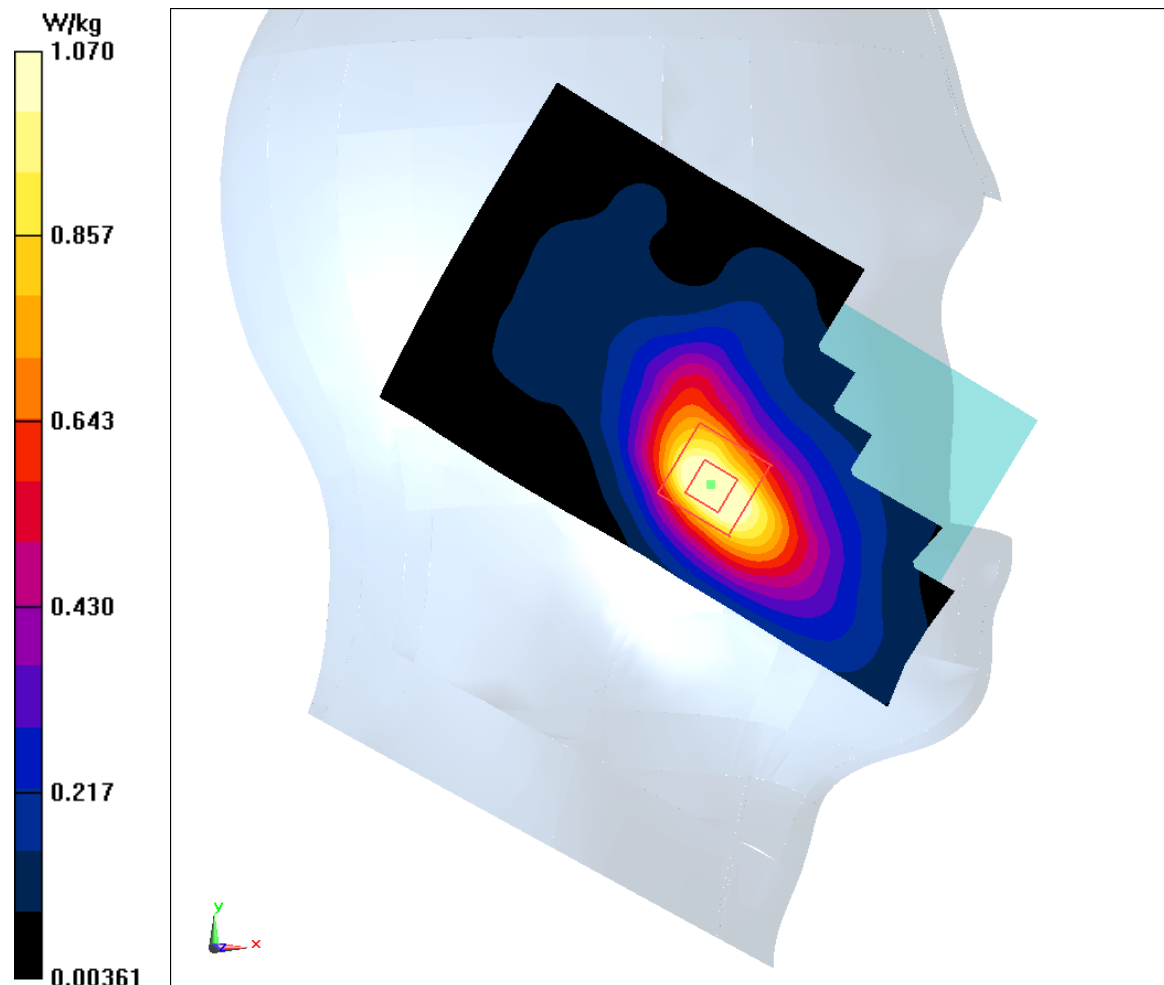
Fig.13 LTE Band7
