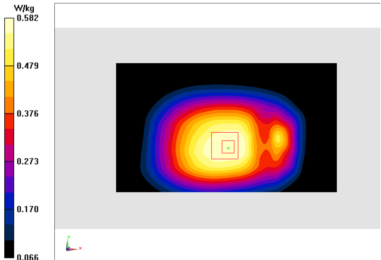
Fig.6 WCDMA 850
