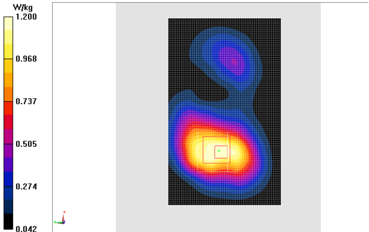
Fig.8 WCDMA1900
