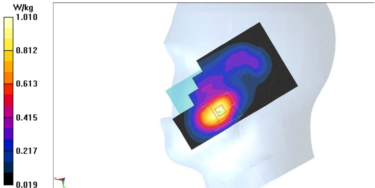
Fig.7 WCDMA1900
