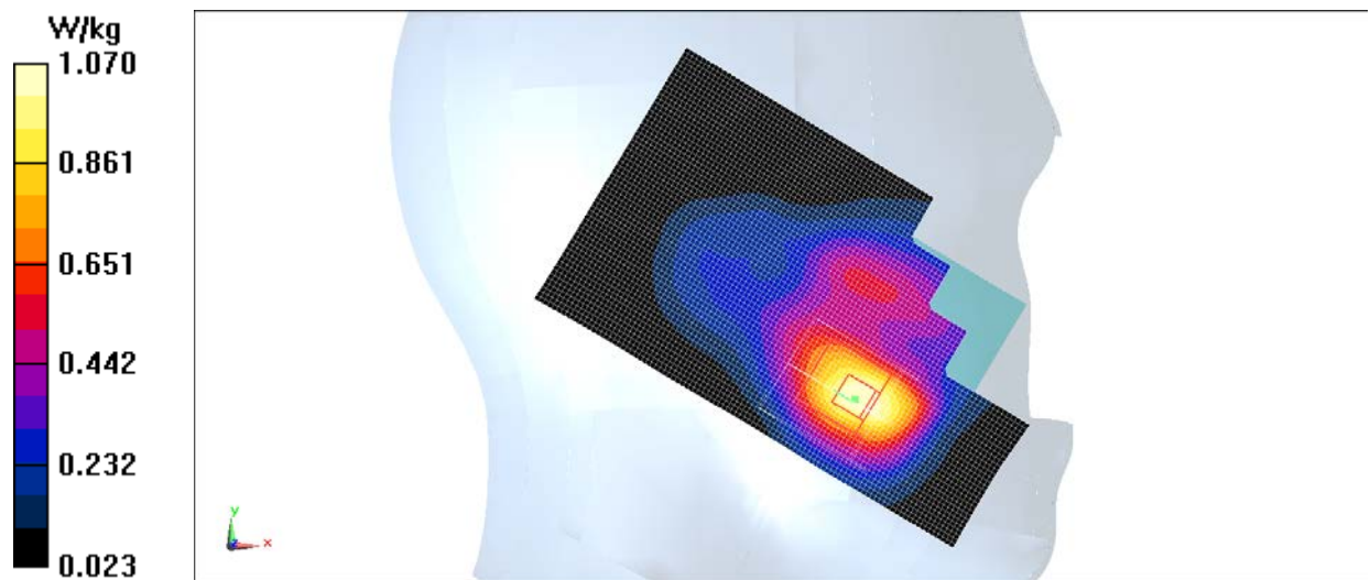
Fig.7 WCDMA1700
