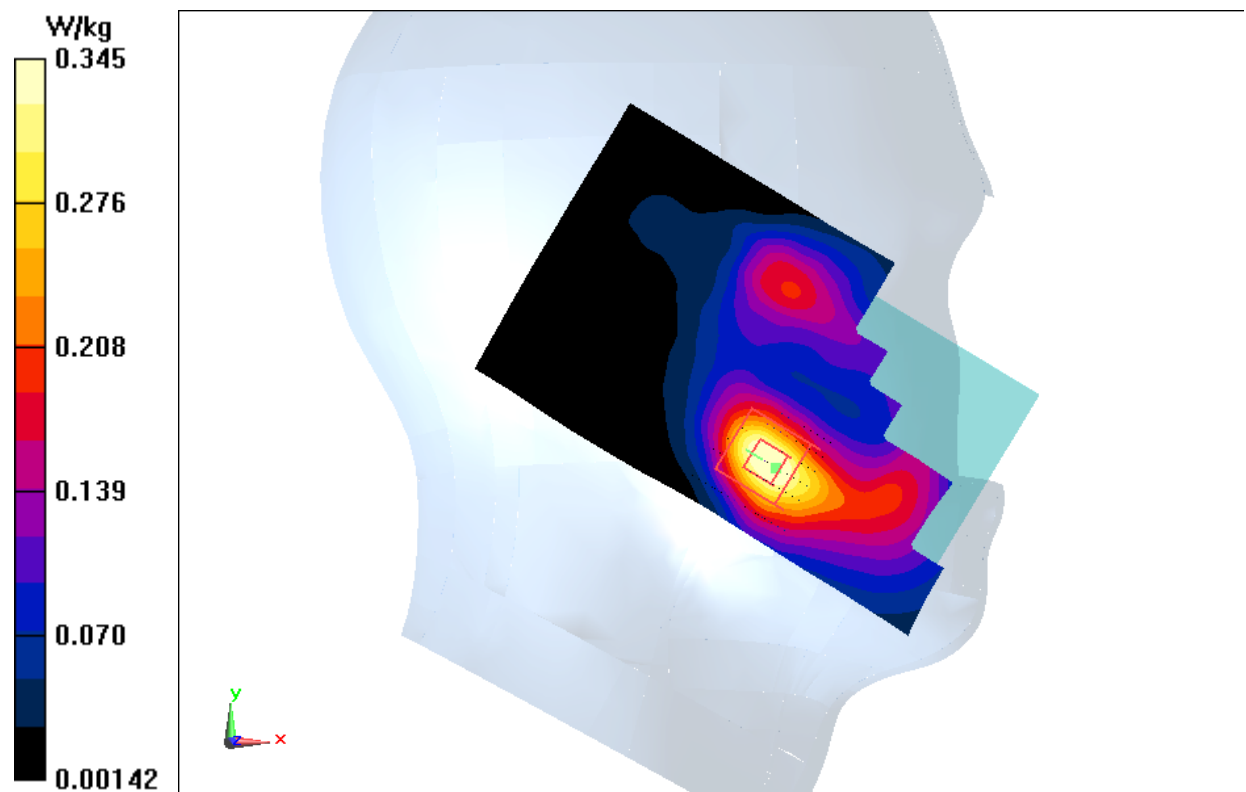
Fig.9 LTE Band7
