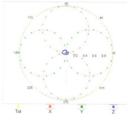
f=600 MHz, TEM, 0^\circ
