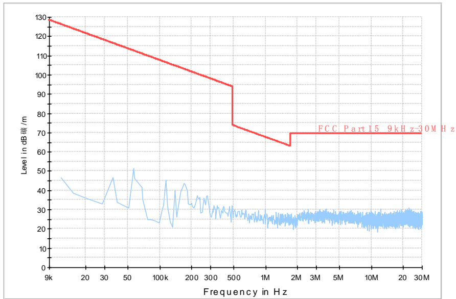
RE_9kHz-30MHz
