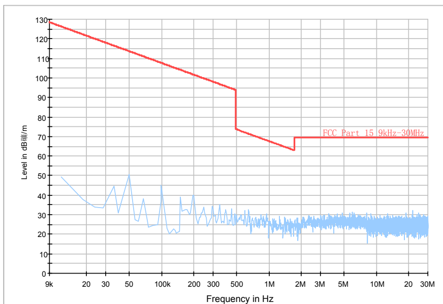
RE_9kHz-30MHz
