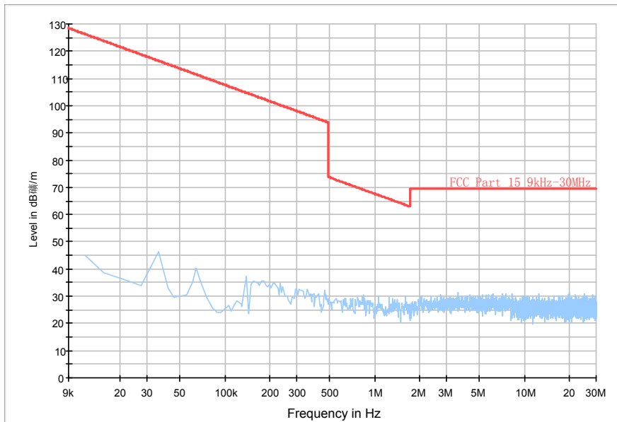
RE_9kHz-30MHz
