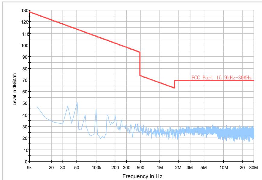
RE_9kHz-30MHz
