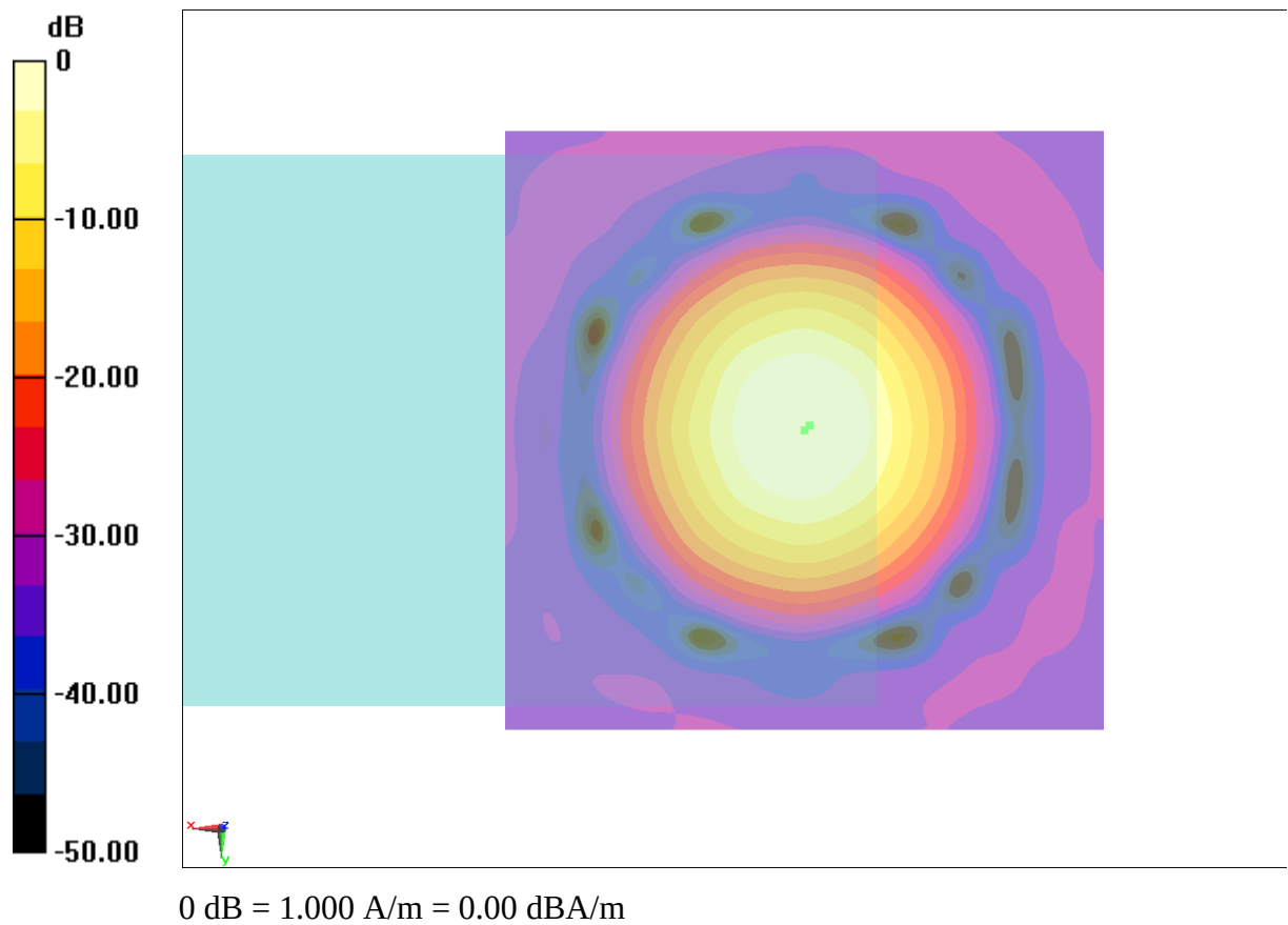
Fig B.8 T-Coil WCDMA 1900
