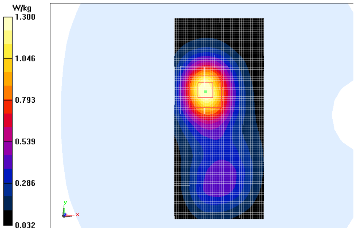
Fig.8 WCDMA1900 CH9538
