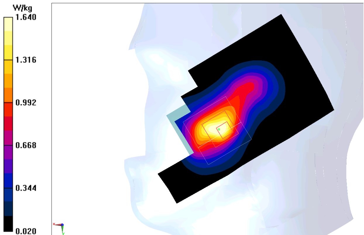
Fig.7 WCDMA1900 CH9538
