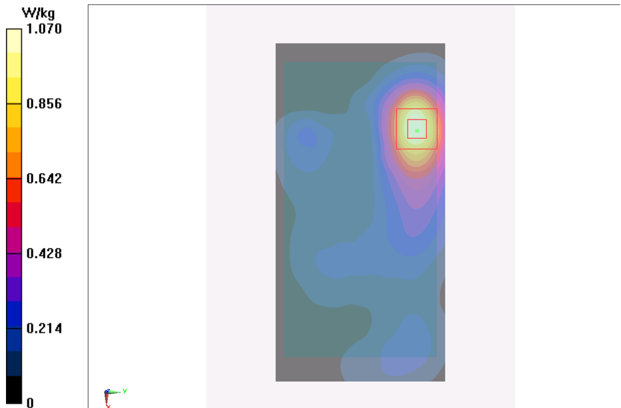
Fig.14 LTE Band7 CH21350
