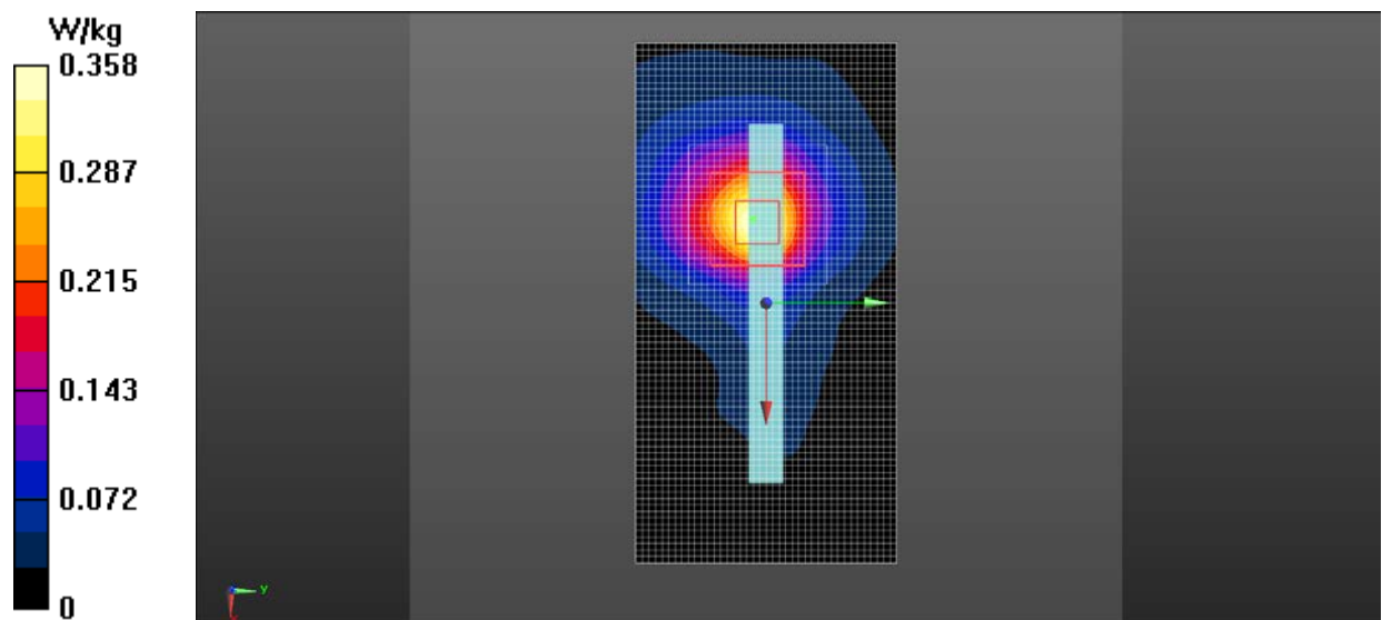
Fig.18 5GHz CH52
