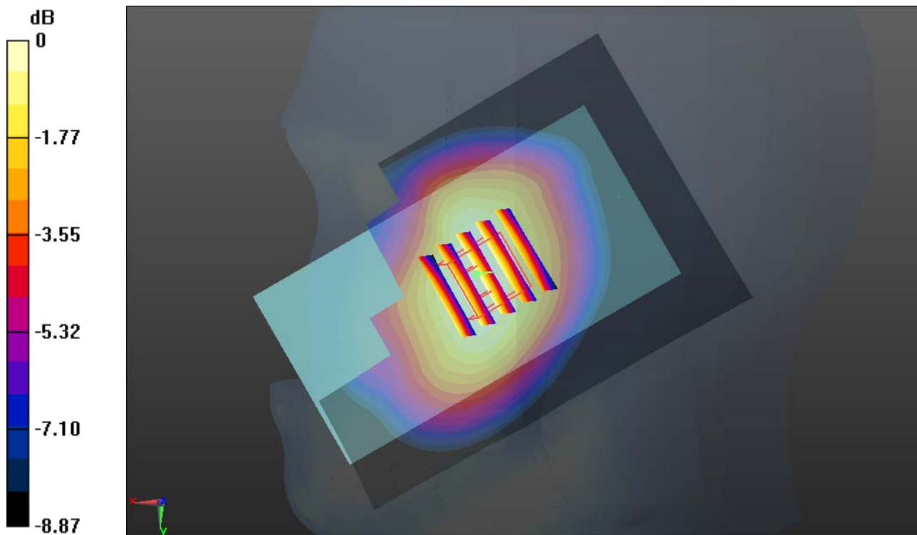
0 dB = 0.220mW/g
