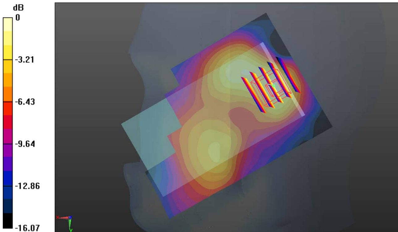
0 dB = 0.100\text{mW/g}
