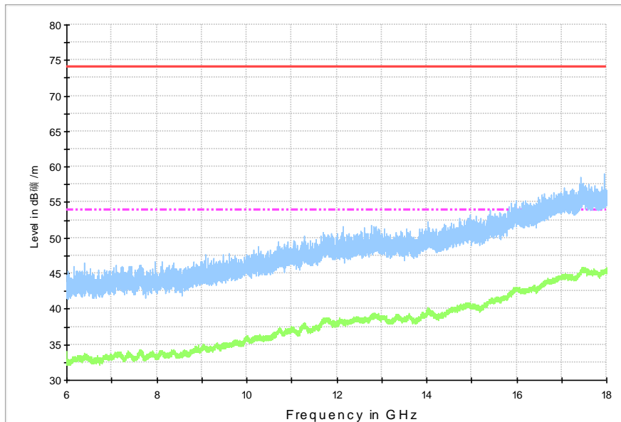
RE - 6GHz-18GHz
