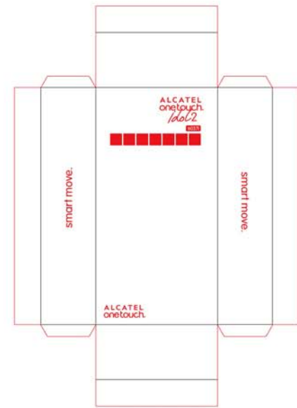
bottom side 179*92*41.5mm
