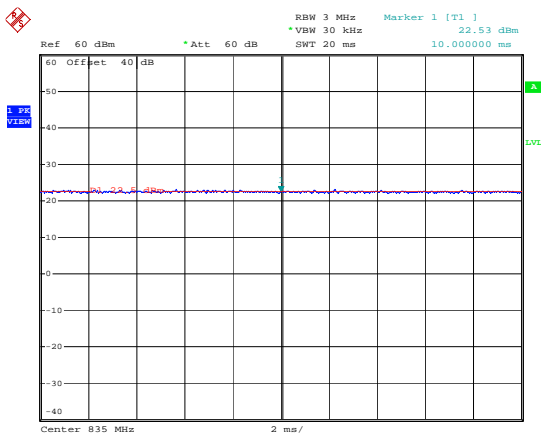
835MHz - WCDMA
