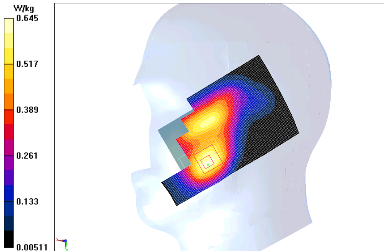
Fig.I.7 WCDMA1900 CH9538
