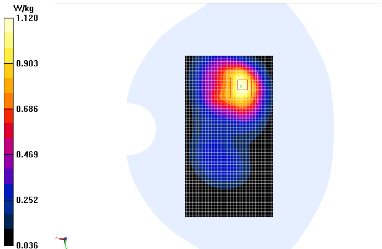
Fig.I.8 WCDMA1900 CH9262
