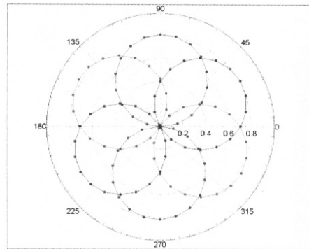
f=1800 MHz,R22
