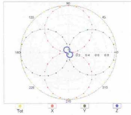
f=2500 MHz,R22,0°
