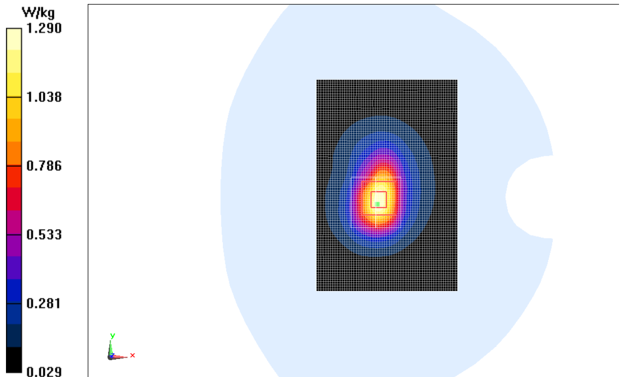
Fig.8 WCDMA1900 CH9400
