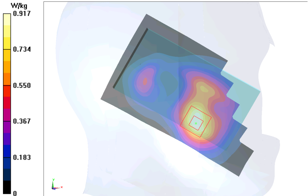
Fig.7 WCDMA1900 CH9538
