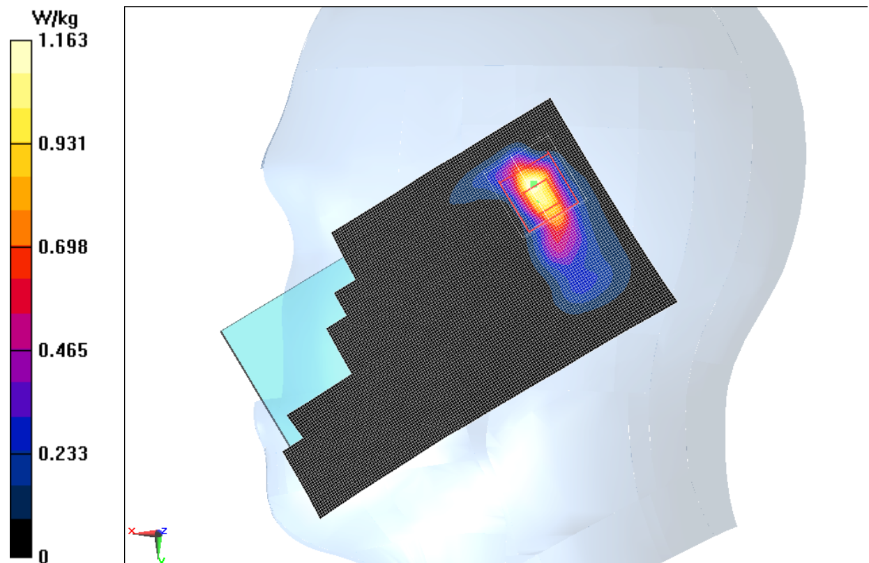
Fig.11 5GHz CH36
